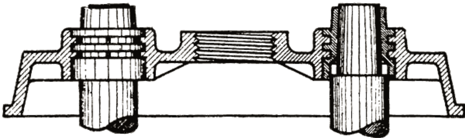
Fig. 11. U. S. L. Cover
