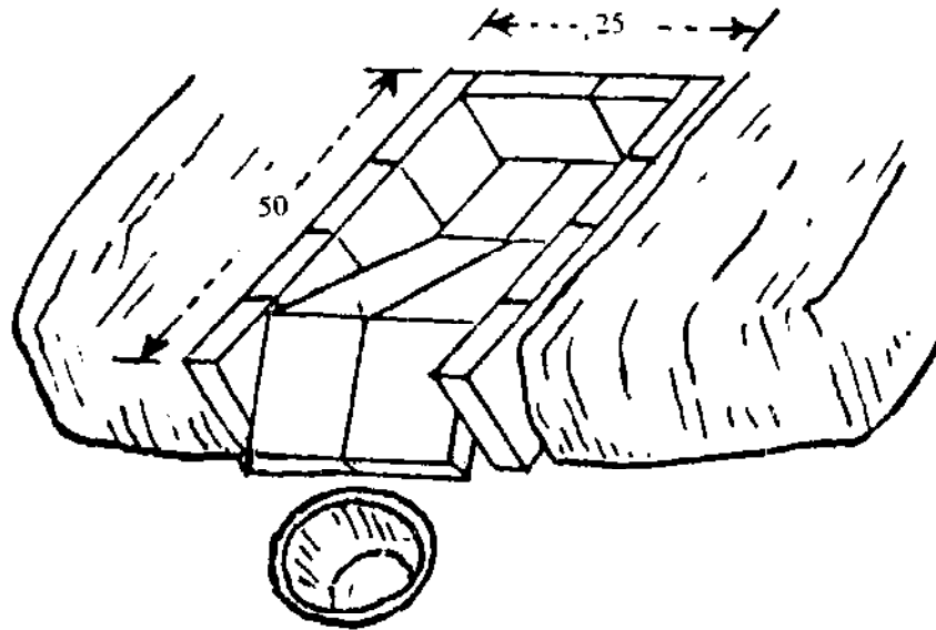
Fig. 7. Ridge toilet (2).
