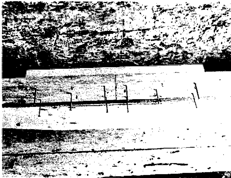
Fig. 145 Poser 10 autres clous sur les bordes, disposés selon photo, enfoncer et retourner. lorsqu'on aura plus d'un joint à faire dans les bordes, le deuxième sera à l'autre bout du bateau et alterné ainsi de suite Fig. 145 Place 10 more nails on the planking as indicated on the photo, hammer in and turn ends, when there is more than one joint to be made in the planking, the second joint should be at the other end of the canoe. Joints should always be alternated this way
