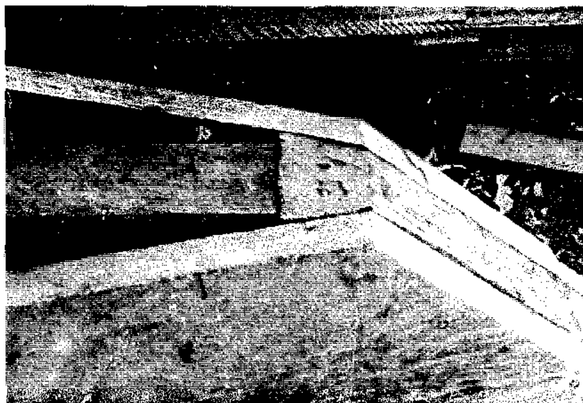
Fig.105 Ajuster le bouchain à effleurer le haut de l'étrave
