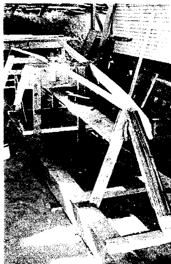
Fig.104 Serrer le bouchain en position contre la première membrure
