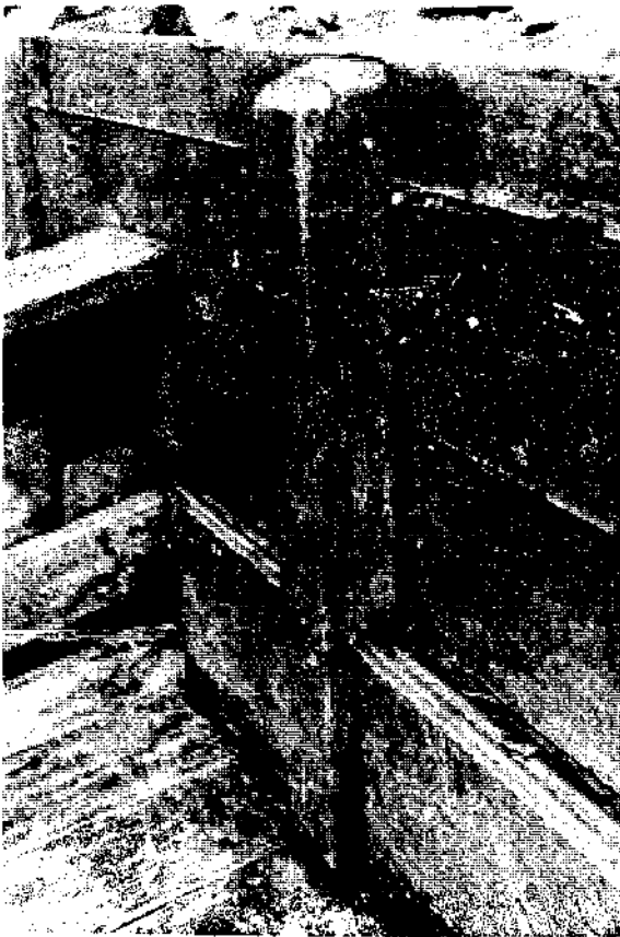
Fig.119 Si les longueurs disponibles ne suffisaient pas, pour disposer le joint entre deux renforts comme ci-haut on fera un joint normal. On devra fixer le renfort sur le joint et ajouter du côté des bordés une pièce de même épaisseur que le joint
