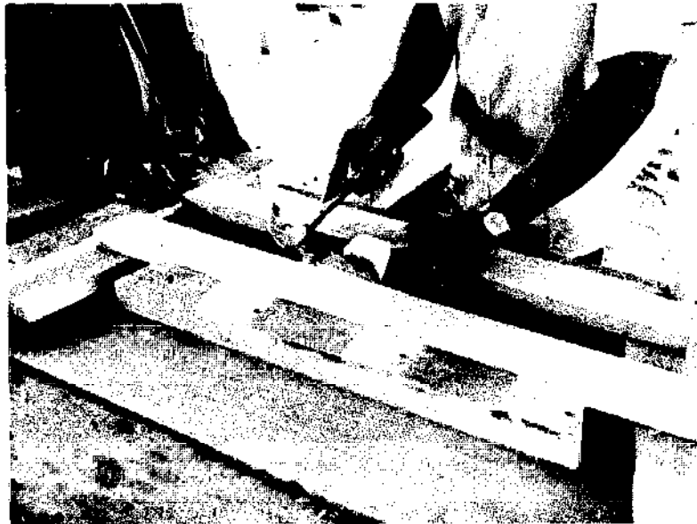
Fig.72 Coincer les deux traverses par un bloc et un coin. Taper doucement sur les bouts de côtés de membrures pour s'assurer qu'ils buttent contre le gabarit. Avec le gabarit troué de traverses marquer les trous de vis sur chaque traverse Fig.72 Tighten the two braces with a block and wedge. Tap lightly on upper ends of frame sides to ensure that bottom edges touch pattern blocks. Mark screw holes on both braces with pattern
