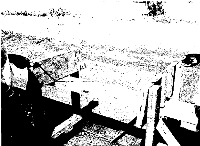
Fig.62 Cette mesure doit être la même à 2 mm près lorsque faite aux deux autres coins des planches
