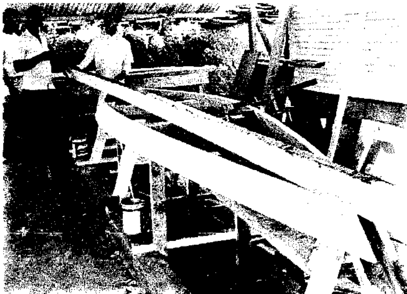
Fig.132 Appliquer le produit d'étanchéité sur une rive de la planche
