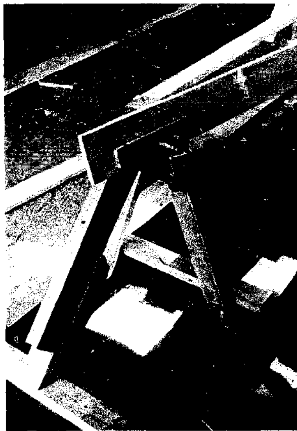
Fig.102 On le maintiendra par un serre-joint dont la vis est calée d'un bloc pour ne pas abîmer le bouchain. On pliera le bouchain jusqu'à l'autre étrave pour s'assurer de sa longueur suffisante. Si la planche est trop courte on y fera un joint. (Voir détail au chapitre joint.) On fera de même pour l'autre bouchain. Appliquer le produit d'étanchéité sur les deux côtés de l'étrave. Reposer le bouchain en prenant soin que le doigt du serre-joint appuie contre le porte-étrave et l'arête de l'étrave
