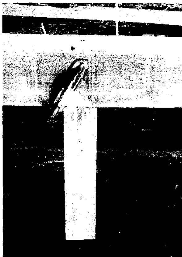
Fig.126 Il est préférable que la vis de la presse soit à l'intérieur de la pirogue et le doigt de la presse centré à l'extérieur du bouchain pour pouvoir clouer de chaque côté Fig.126 The clamp screw should be on the inside of the canoe to ease nailing, the clamp finger at the centre of the plank to permit nailing on each side of it
