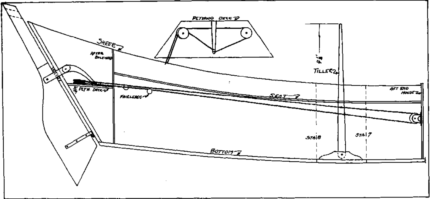
Steering rig.
