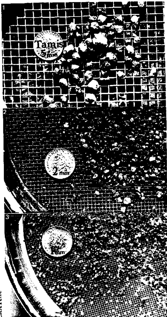
FIGURE 242 : LES REFUS DOIVENT ETRE TRES PROPRES AVANT D'ETRE ETUVES ET PESES
