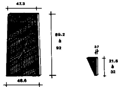
FIGURE 12 : FOND DE BANCHE ET COIN
