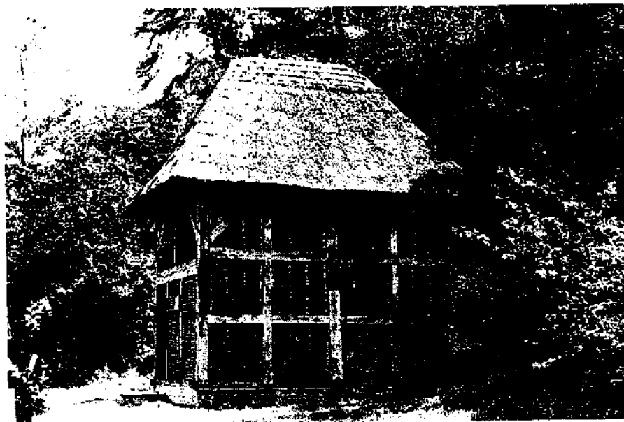
FIGURE 293 : ▶ « CATHERINGTON TREAD WHEEL » XI e SIÈCLE (MUSÉE EN PLEIN AIR DE SINGLETON) CETTE PETITE MAISON ABRITTE UNE ROUE DANS LAQUELLE MARCHAIT UN HOMME POUR FAIRE REMONTER L'EAU D'UN PUY. ELLE N'A JAMAIS ÉTÉ ENDUITE DE TERRE, CHOSE COURANTE À L'ÉPOQUE
