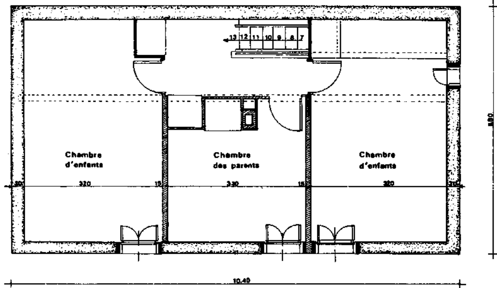
FIGURE 111 : ETAGE
