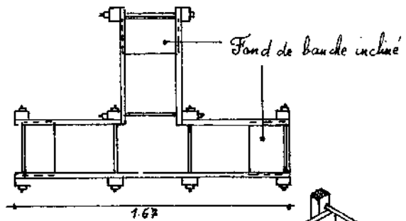
Banche roulante
