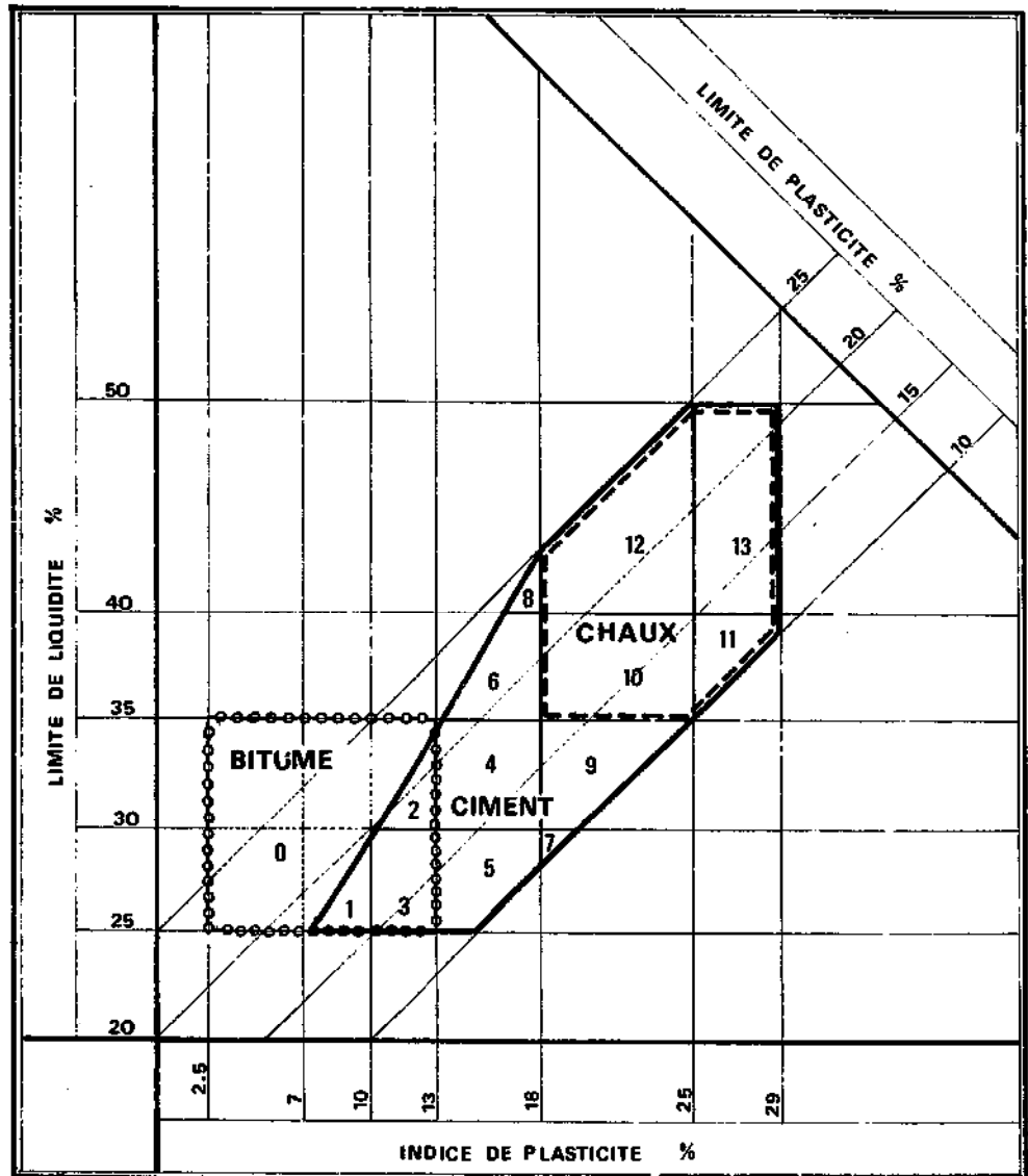
▲ FIGURE 281 : FUSEAU DE STABILISATION POUR LE CIMENT, LA CHAUX, LE BITUME, SEULS LES ELEMENTS FINS (INFÉRIEURS A 0,5 mm) SONT PRIS EN CONSIDÉRATION
