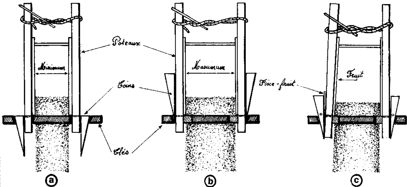
FIGURE 14 : (a) et (b) L'ECARTEMENT DES BANCHES VARIE EN FONCTION DE L'ENFONCEMENT DES COINS - (c) MANIERE DE MONTER LE FRUIT DU MUR
