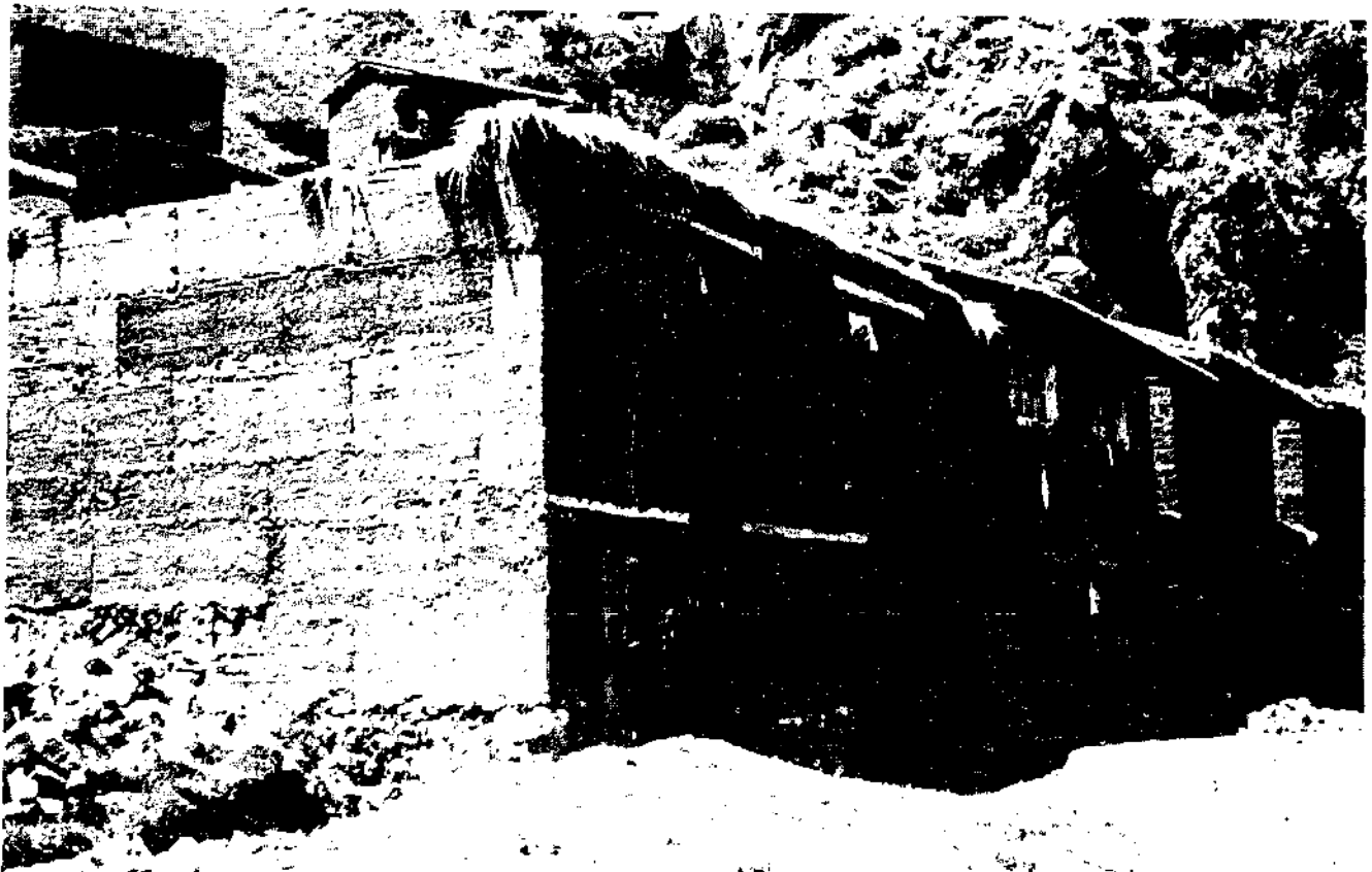
5 - On la dame avec le pisoir (fig. 61). On utilise parfois un pisoir à deux manches encadrant un gros morceau de bois. L'installation de la banche sur le mur demande 20 minutes et son remplissage, par trois hommes et deux enfants de 40 à 50
