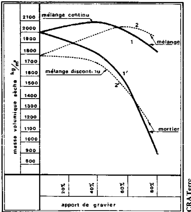
FIGURE 271 : COMPACTITES D'UN MELANGE MORTIER-GRANIER
