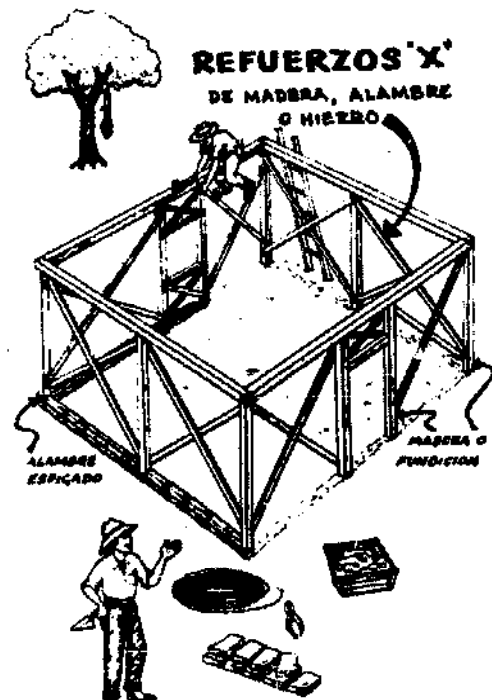
FIGURE 192 : STRUCTURE PARASISMIQUE GUATEMALA. EN HAUT : RENFORCEMENTS EN « X » EN EN BOIS, FIL DE FER, OU FER A GAUCHE : FIL DE FER BARBELE A DROITE : BOIS OU BETON
