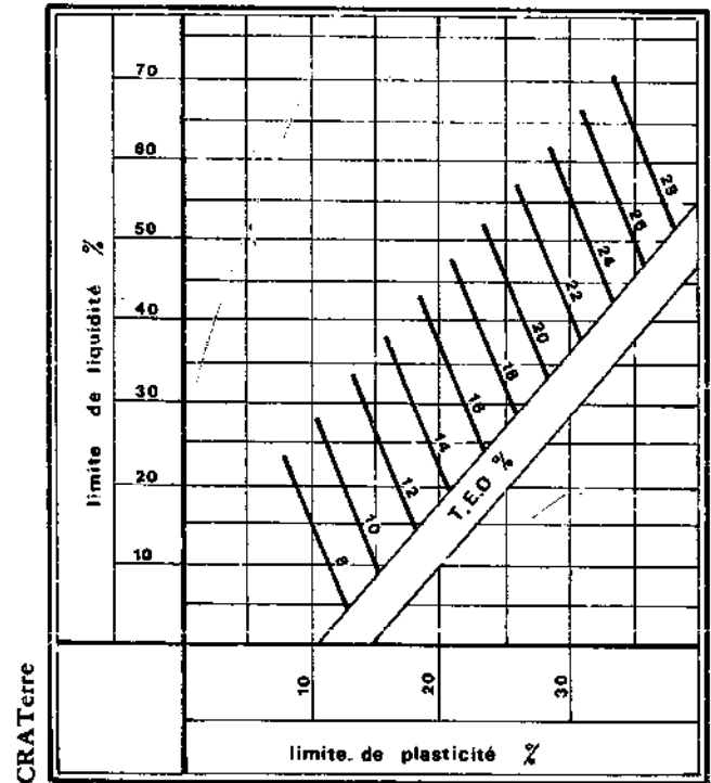
FIGURE 273 : LIMITES D'ATTERBERG ET DENSITE
