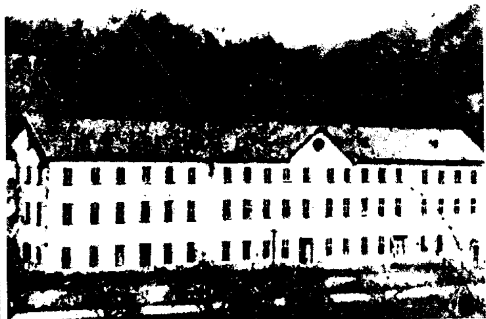
FIGURE 66 : FABRIQUE DE CERAMIQUE (PISE) BATIE PAR WIMPF AU DEBUT DU XIX e SIECLE. APRES 45 ANS D'ABANDON TOTAL (TOIT ET VITRES BRISES), CETTE CONSTRUCTION CONSERVE EN 1920 DES MURS ET DES ENDUITS INTACTS. IL A FALLU DETRUIRE A LA DYNAMITE CETTE USINE EN PISE (STABILISE PAR LA CHALEUR DES FOURS) QUI N'EXISTE PLUS DE NOS JOURS.
