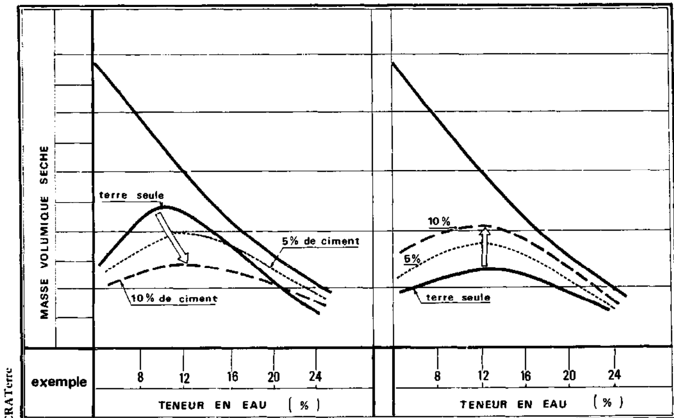
FIGURE 283 : INFLUENCE D'ADJONCTION DE CIMENT SUR LA MASSE VOLUMIQUE SECHE
