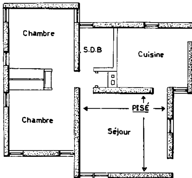
FIGURE 94 : EXEMPLE DE CONSTRUCTION ARCHITECTURALE ELIMINANT LES ANGLES EN PISÉ (HIBBEN)
