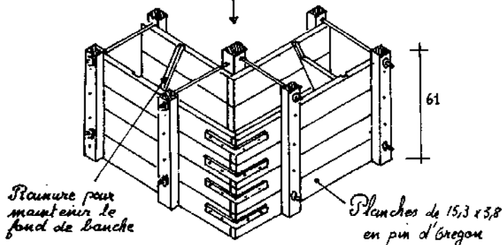
Banche d'angle
