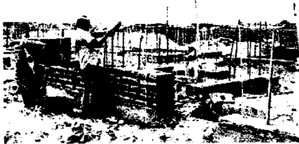
FIGURE 207 - ELÉVATION DU MUR, LES BRIQUES TROUÉES SONT ENFILÉES SUR LES ROSEAUX
