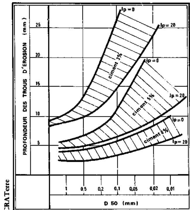
FIGURE 287 : RESISTANCE A LA PLUIE ET DIAMETRE MOYEN DES GRAINS POUR DIVERSES TENEURS EN CIMENT
