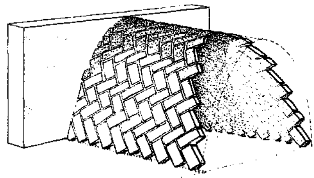
FIGURE 307 : APPAREILLAGE EN EPIS (OU EN CHEVRON)
