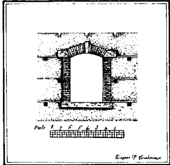
▲ FIGURE 31 32 : LES ENCADREMENTS DES PORTES ET DES FENETRES SE FONT SOUVENT EN MAÇONNERIE, EN BRIQUES OU EN BOIS. DES CADRES PLACÉS DANS LA BANCHE, SOLIDEMENT ET AYÉS, ET SERVANT DE « RÉSERVATION » LORS DU D'AMAGEMENT TIEN AIENT PARFOIS LIEU DE CHASSIS.
