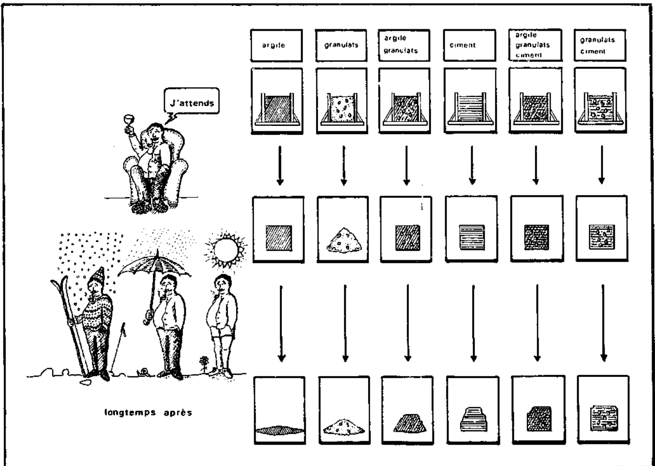
FIGURE 267 : COMPORTEMENT DE DIFFERENTS MELANGES - JUSTE APRES DEMOULAGE (COHESION) - APRES QUELQUES ANNEES (RESISTANCE AUX INTEMPERIES - EAU - GEL - DESSICATION)
