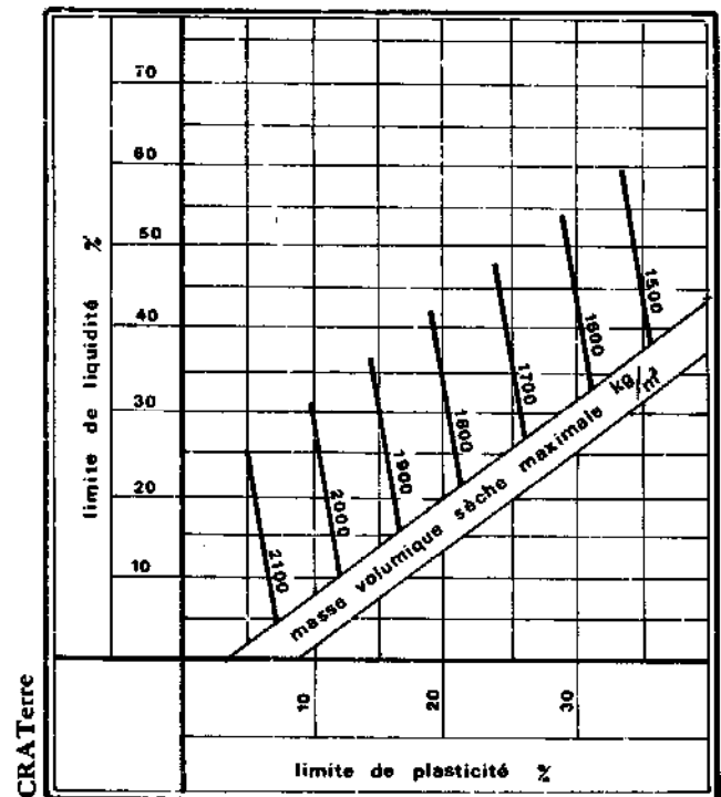
FIGURE 273 : LIMITES D'ATTERBERG ET DENSITE
