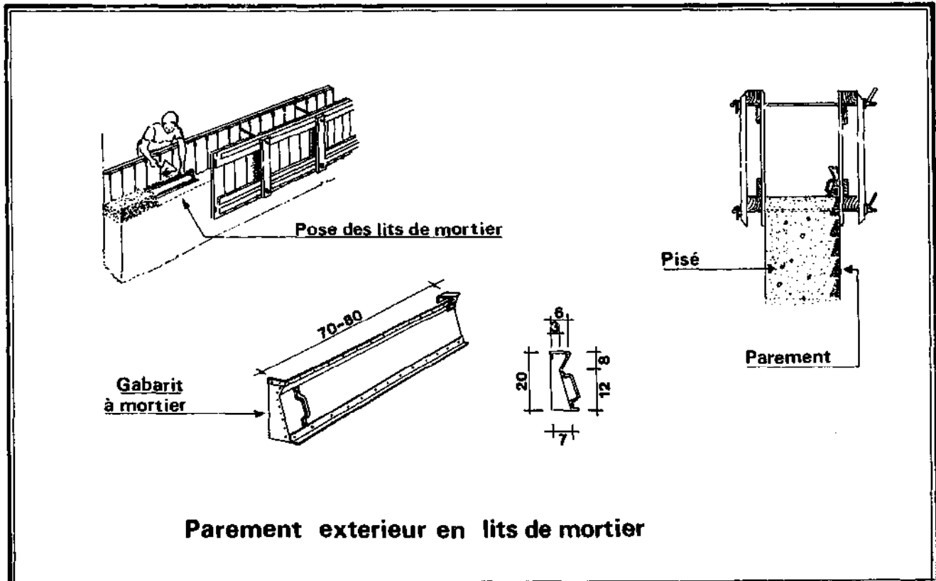
FIGURE 325 : PAREMENT EXTERIEUR EN LITS DE MORTIER
