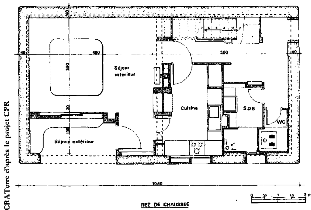
FIGURE 110 : REZ-DE-CHAUSSEE
