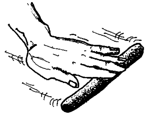
FIGURE 160 : TEST POUR VÉRIFIER L'APTITUDE DE LA TERRE À LA FABRICATION DE L'ADOBE
