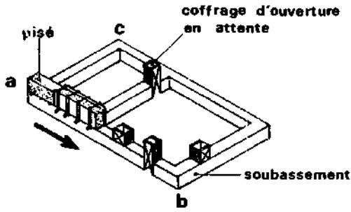
1 ère ASSISE
