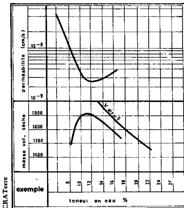
FIGURE 276 : PERMEABILITE ET T.E.O.
