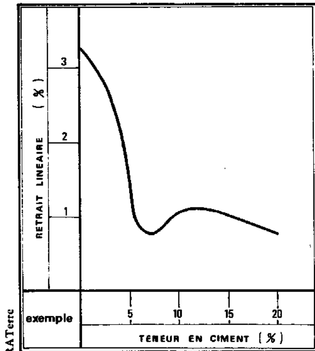
FIGURE 286 : VARIATION DU RETRAIT AVEC LA TENEUR EN CIMENT
