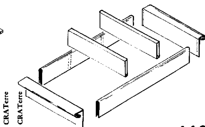
2 - MOULE EN TOLE POUR TROIS BLOCS DE 19 x 39 x 9 cm
