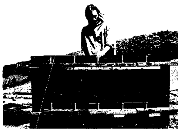
FIGURE 97 : BANCHE ARTICULEE PERMETTANT DES MURS COURBES AINSI QUE DES POTEAUX - POSITION RECTILIGNE (LE PIN, 1975)
