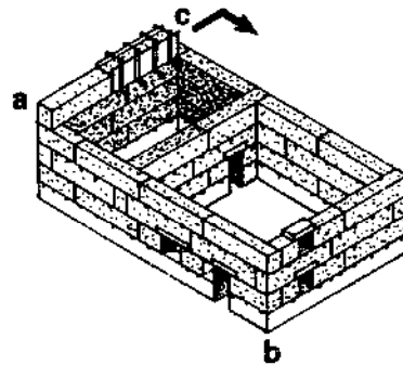
4 ème ASSISE etc...
