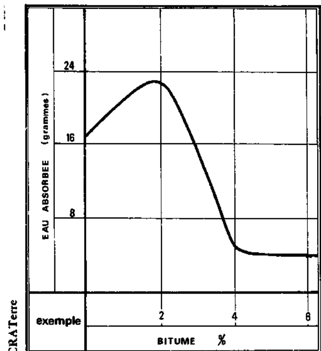
FIGURE 290 : ESSAI D'ABSORPTION
