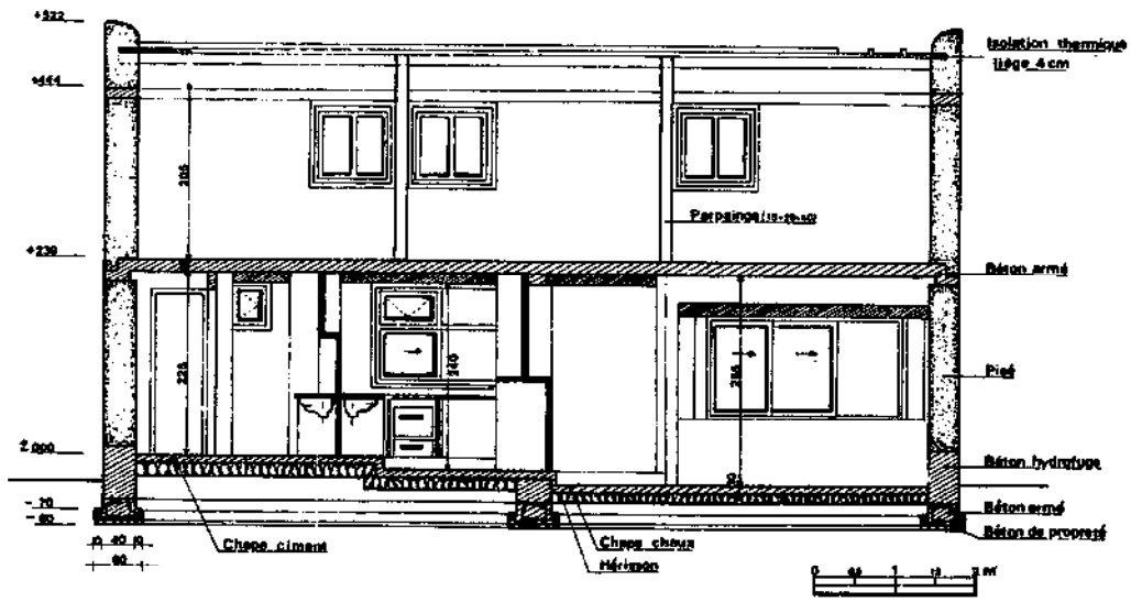
FIGURE 113 : COUPE LONGITUDINALE
