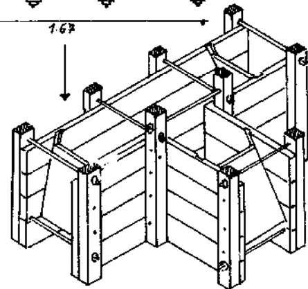
Banche pour mur de refend
