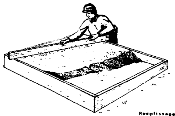
FIGURE 176 : ADOBE DECOUPEE
