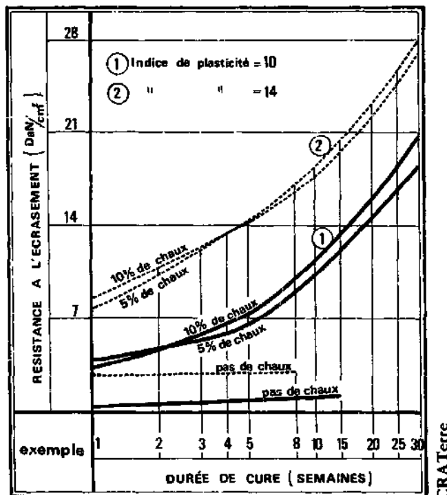
FIGURE 288 : TEMPS DE CURE ET RESISTANCE
