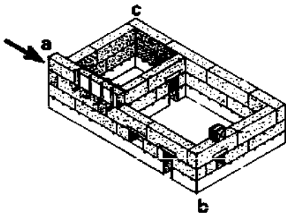
3 ème ASSISE
