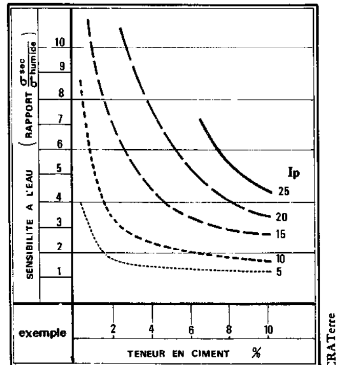
FIGURE 285 : SENSIBILITE A L'EAU SELON LA TENEUR EN CIMENT ET I_p POUR UN MEME COMPACTAGE
