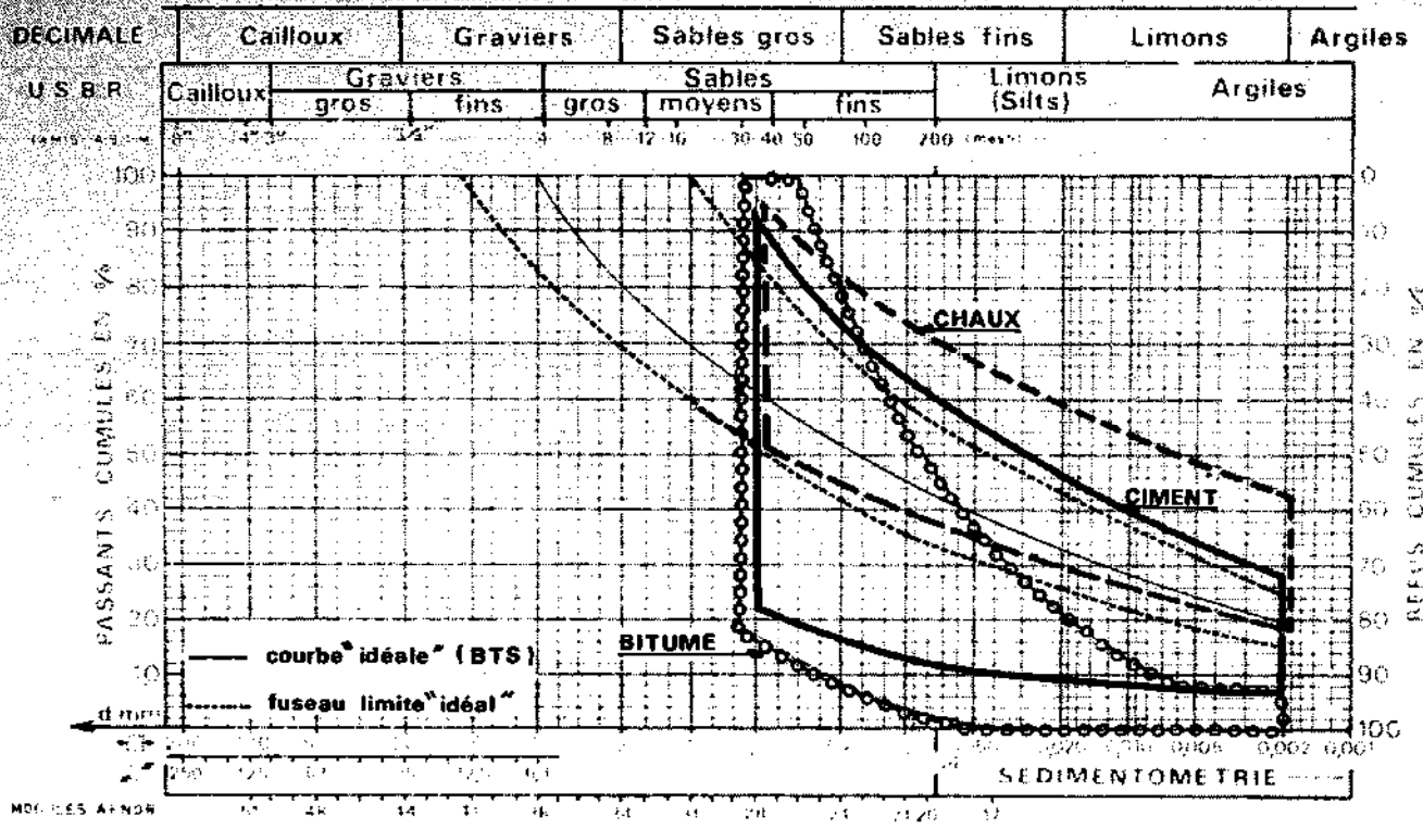
▲ FIGURE 281 : FUSEAU DE STABILISATION POUR LE CIMENT, LA CHAUX, LE BITUME, SEULS LES ELEMENTS FINS (INFÉRIEURS A 0,5 mm) SONT PRIS EN CONSIDÉRATION
