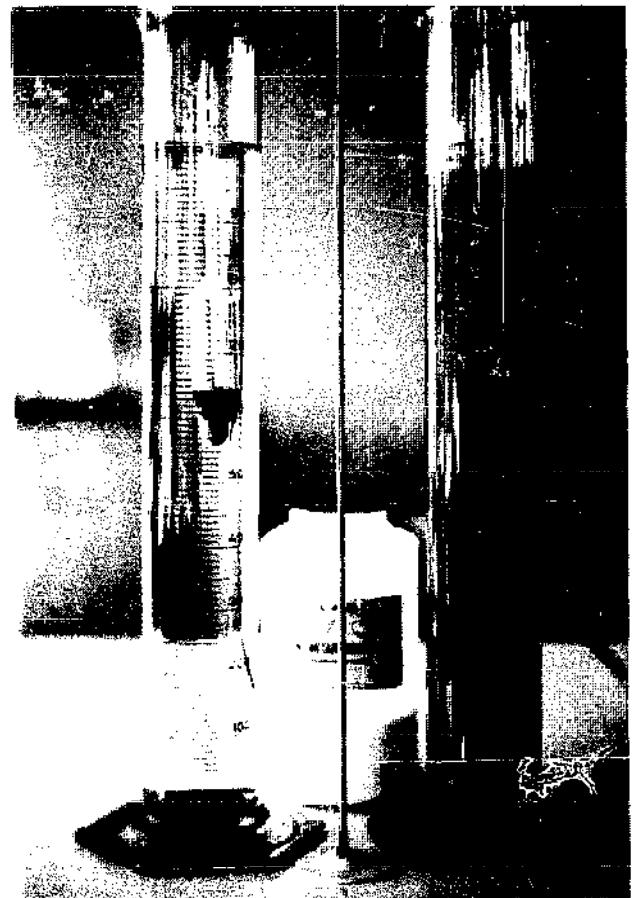
FIGURE 248 : MATERIEL POUR SEDIMENTOMETRIE (1 DENSIMETRE GRADUE DE 995 A 1030 DE FORME TORPILLE, 2 EPROUVETTES DE 1 L, 1 THERMOMETRE, 1 AGITATEUR, DU DEFLOCULANT, 1 FICHE, 1 CHRONOMETRE).
