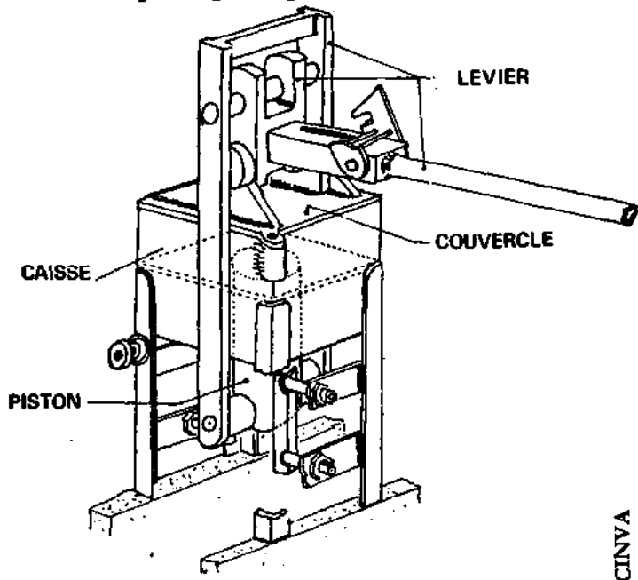
FIGURE 219 : LA PRESSE CINVA-RAM
