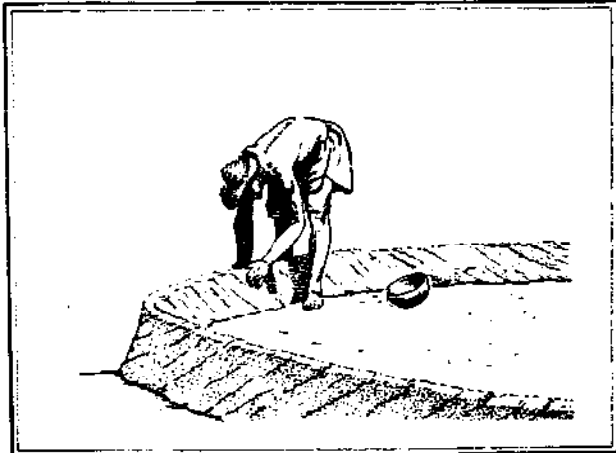
FIGURE 130 : LE MAÇON FAÇONNE A LA MAIN LA PREMIÈRE ASSISE
