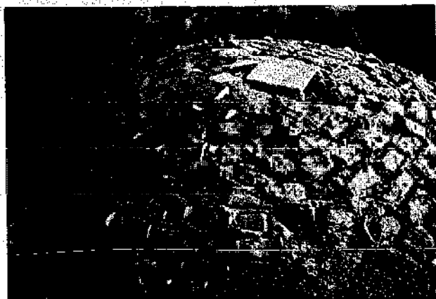
FIGURE 321 : COUPOLE CONSTRUITE SANS COFFRAGE AU NOUVEAU GOURNA (EGYPTE)
