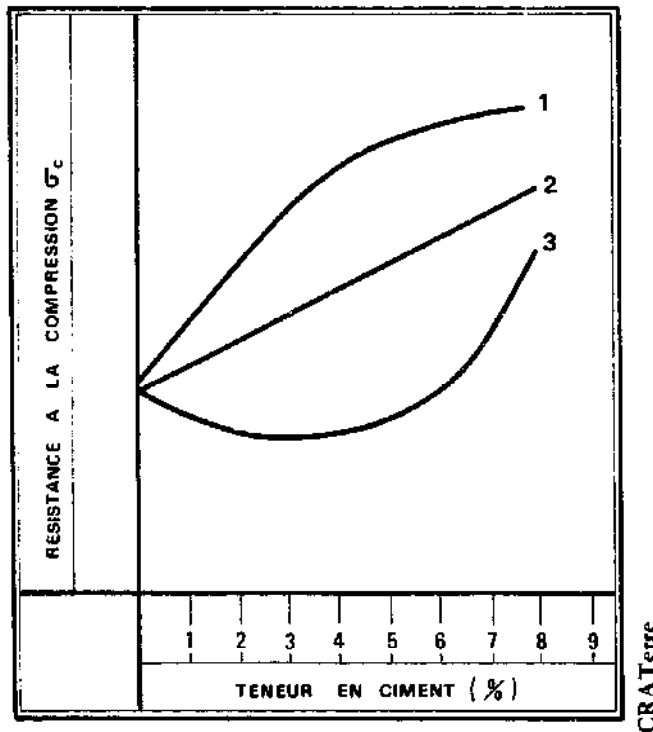
FIGURE 284 : RESISTANCE A LA COMPRESSION ET TENEUR EN CIMENT POUR TROIS SOLS
