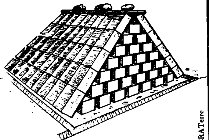
FIGURE 170 : STOCKAGE DE BRIQUES AVEC DRAINAGE (ALLEMAGNE DE L'EST)
