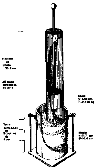
FIGURE 257 : MATÉRIEL POUR L'ESSAI PROCTOR
