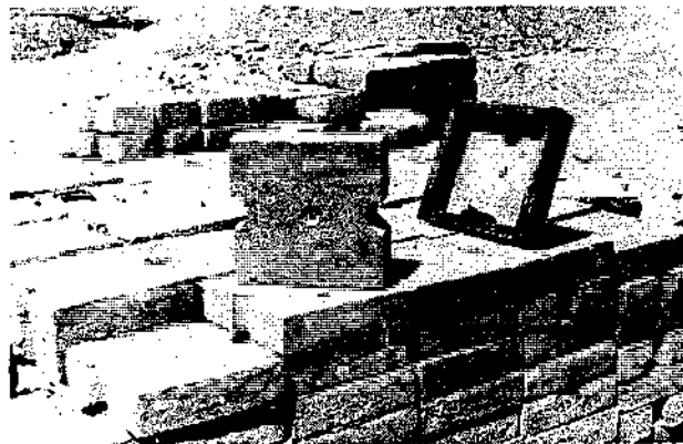
FIGURE 211 : MOULE ET BRIQUE (MAISON EXPERIMENTALE DE LIMA)
