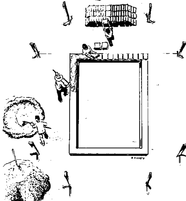
FIGURE 185 : ORGANISATION DU CHANTIER POUR QUATRE PERSONNES
