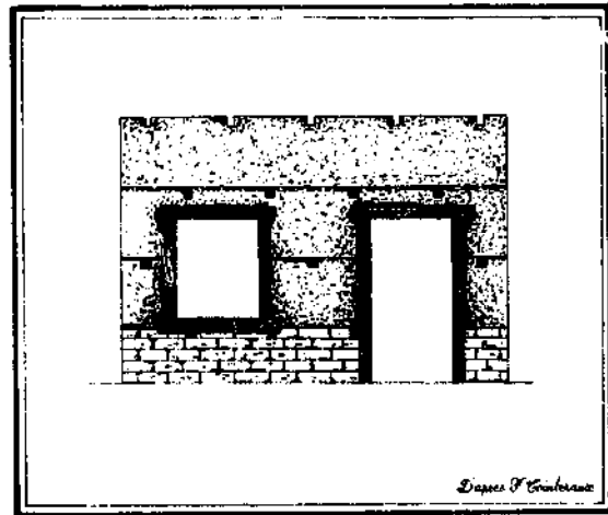
▲ FIGURE 31 32 : LES ENCADREMENTS DES PORTES ET DES FENETRES SE FONT SOUVENT EN MAÇONNERIE, EN BRIQUES OU EN BOIS. DES CADRES PLACÉS DANS LA BANCHE, SOLIDEMENT ET AYÉS, ET SERVANT DE « RÉSERVATION » LORS DU D'AMAGEMENT TIEN AIENT PARFOIS LIEU DE CHASSIS.
