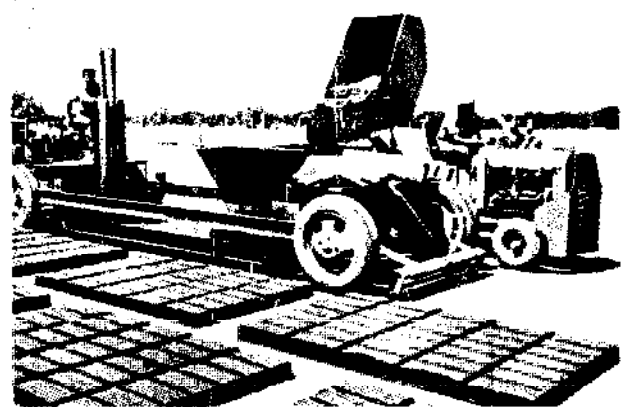
FIGURE 174 : MACHINE A MOULER DE LA « HANS SUMPFF COMPANY » A FRESNO (CALIFORNIE)
