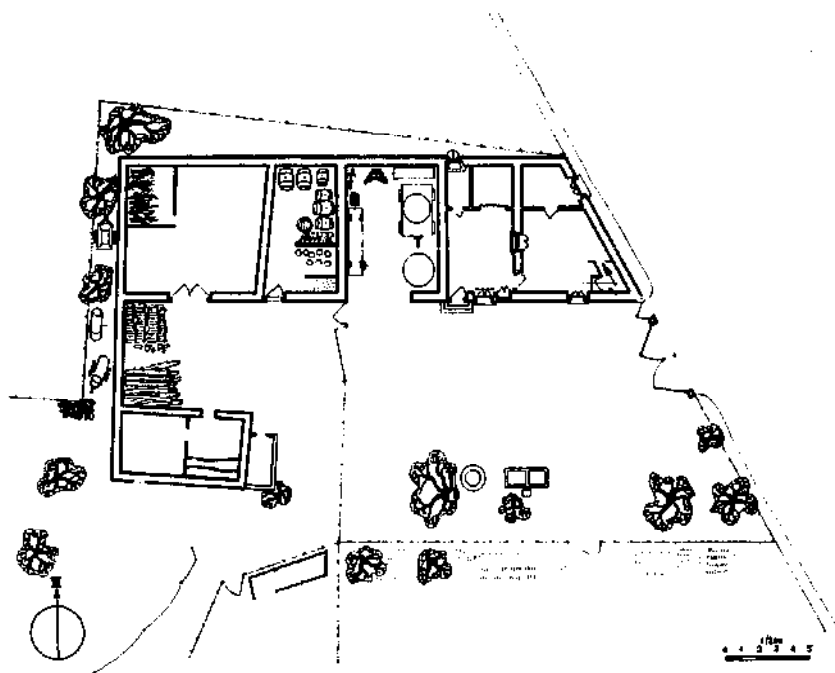
FIGURE 49 : PLAN D'ENSEMBLE
