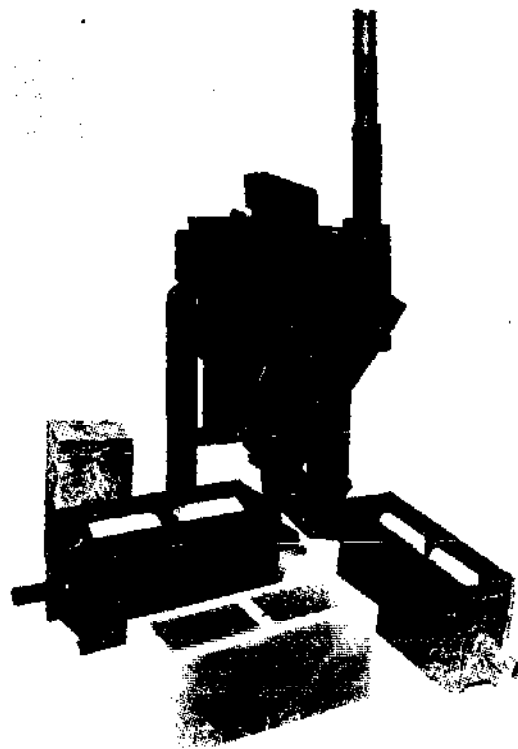
Figure 232 : presse à agglomérés de ciment A.B.I.
