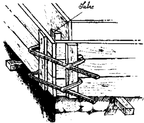
FIGURE 28 : CHAINFREINAGE DE L'ANGLE PAR POSE D'UN « SABRE » DANS L'ANGLE EXTERIEUR DE LA BANCHE
