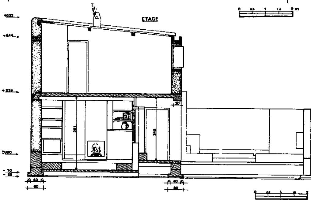
FIGURE 112 : COUPE TRANSVERSALE
