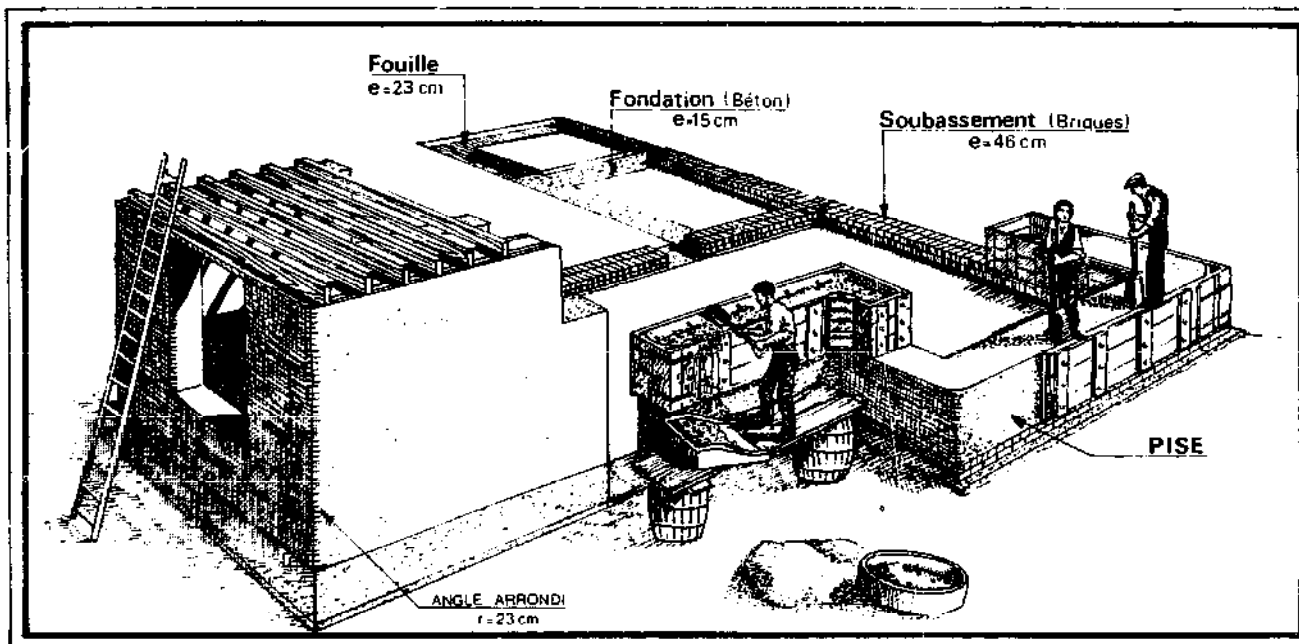
FIGURE 64 : ELEVATION D'UNE MAISON EN PISE EN GRANDE-BRETAGNE
