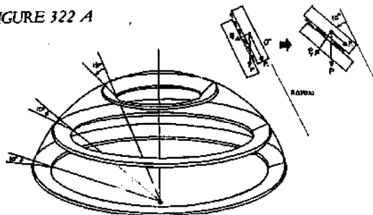
FIGURES 322 : PRINCIPE DE CONSTRUCTION DES COUPOLES SANS COFFRAGE
