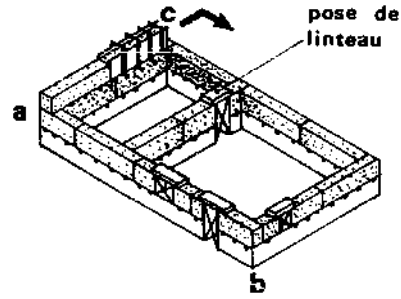
2 ème ASSISE
