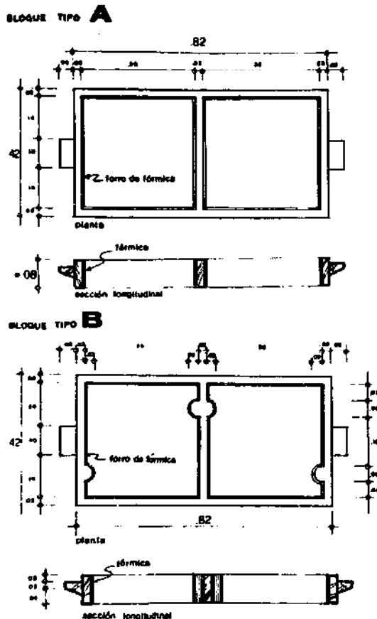
FIGURE 203 : MOULIS UTILISES A CAYALTI
