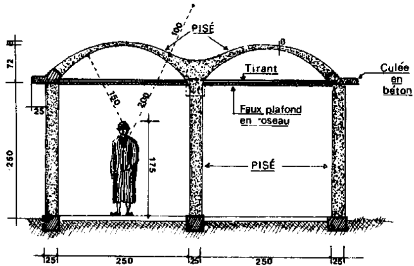
Coupe
