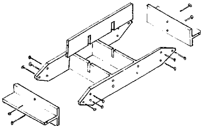
1 - MOULE EN BOIS POUR SIX BRIQUES DE 14 x 29 x 9 cm
