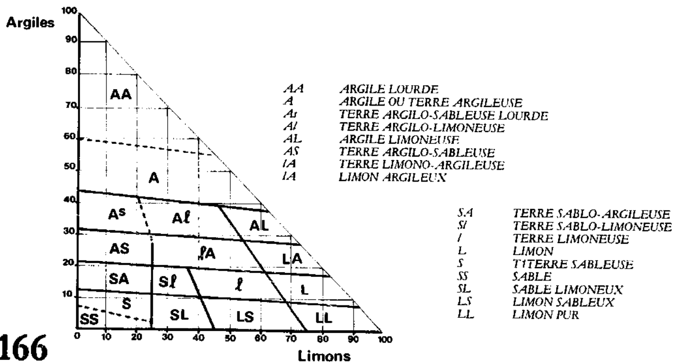
FIGURE 241 bis : TRIANGLE DES TEXTURES DE L'INRA (INSTITUT NATIONAL DE RECHERCHE AGRONOMIQUES)
