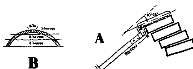
FIGURE 323 : CONSTRUCTION D'UNE COUPOLE SANS CINTRE
