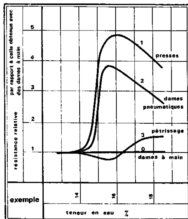
FIGURE 278 : RESISTANCES POUR UNE DEFORMATION DE L'ECHANTILLON DE 5%
