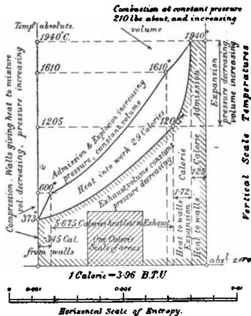
Fig. 117.—Entropy Diagram.
