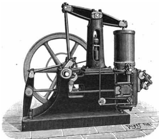
Fig. 165.—Bénier Air Engine. 1886.
