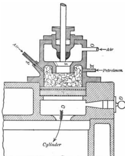
Fig. 127.—Brayton Carburator. 1878.
