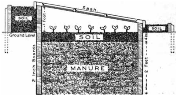
FIG. 27. A simple hotbed. (Erwin.)
