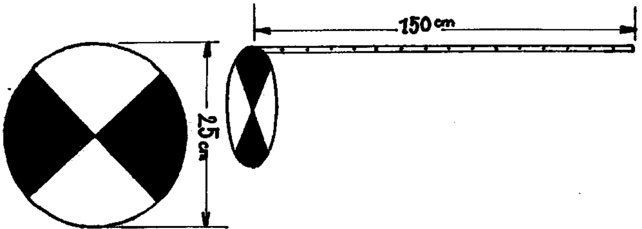
Fig. 12 Secchi disc.
