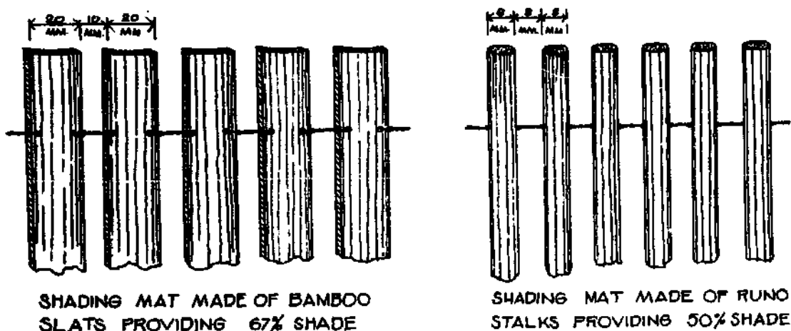
Fig. 36: Shading mats
