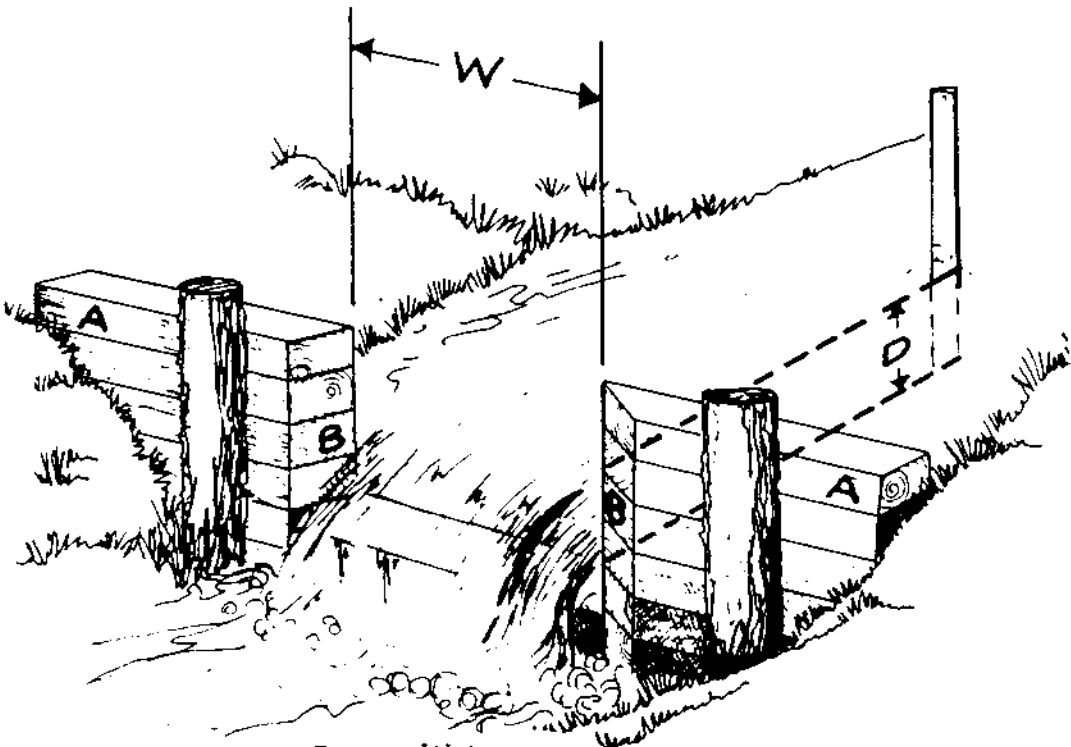
Fig. 1. Weir
