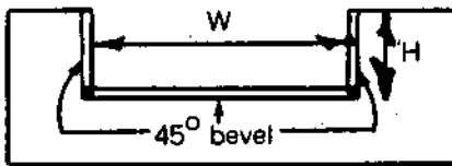
FIG. 1A WEIR
