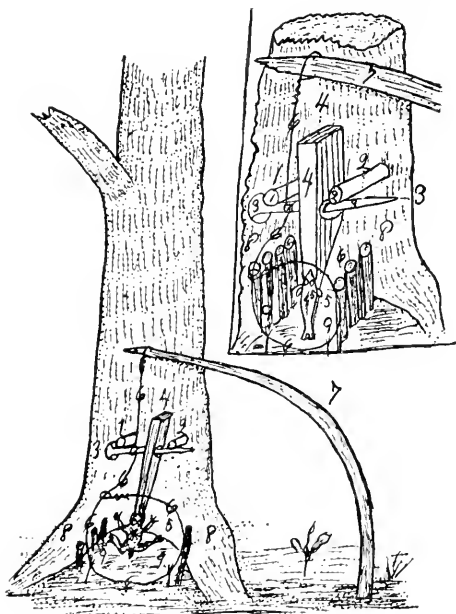
BAIT SET SNARE.
