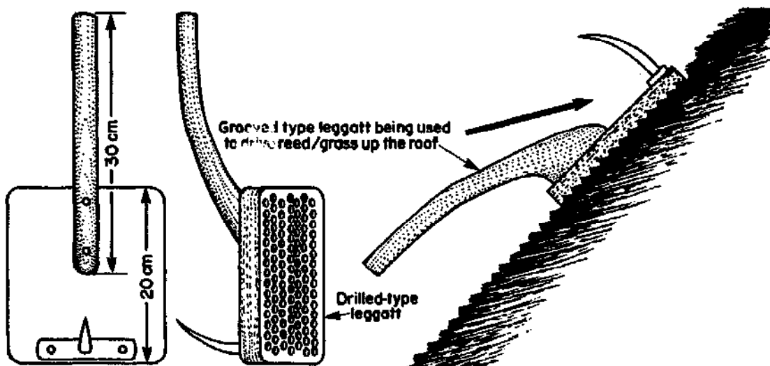
Fig. 4:7 Leggatts.
