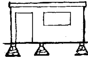
En terreno malo o regular las bases de los cimientos son más anchas.
