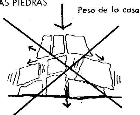
Cimiento incorrecto y peligroso
