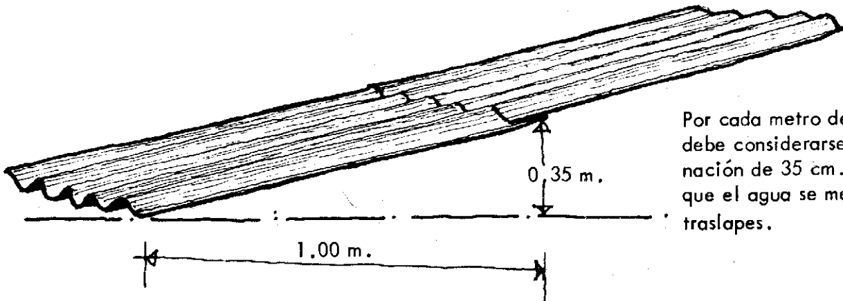
TRASLAPES
