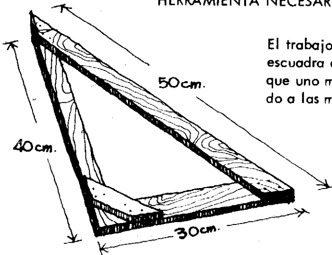
Escuadra de madera.
