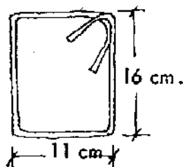
Estriba de alambón
