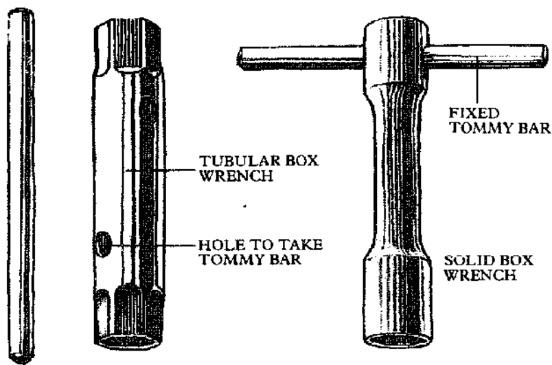
TOMMY BAR
