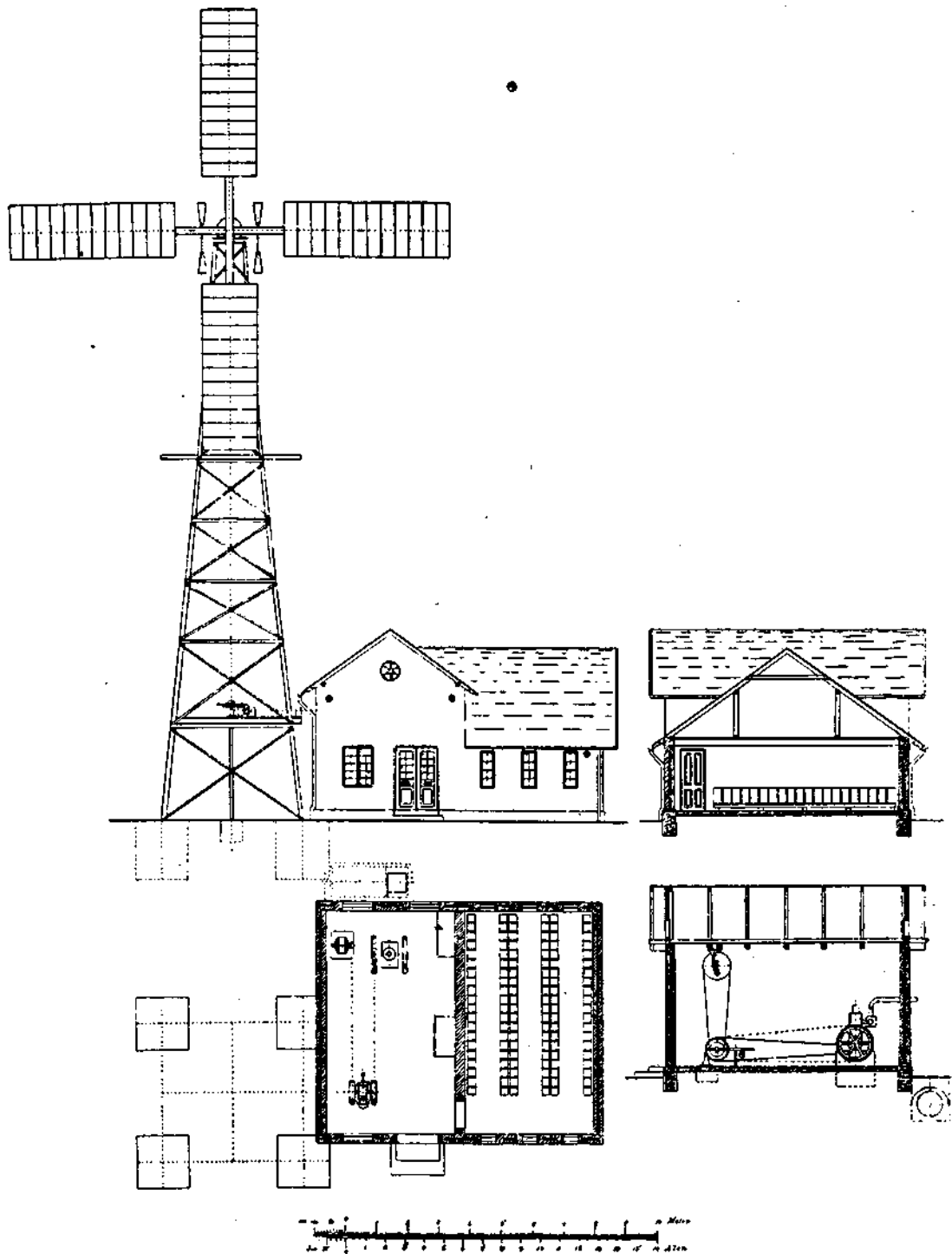
Fig. 3. Mølle med Reservekraft.
