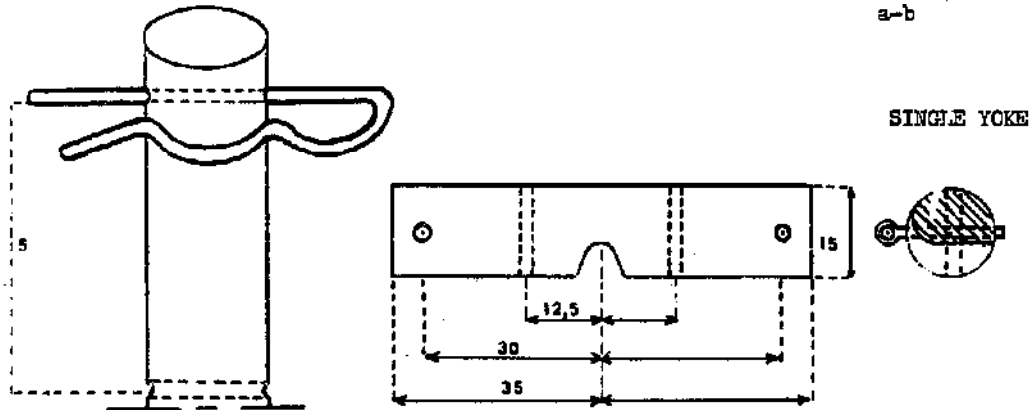
Fig. 38 - LONG YOKE
