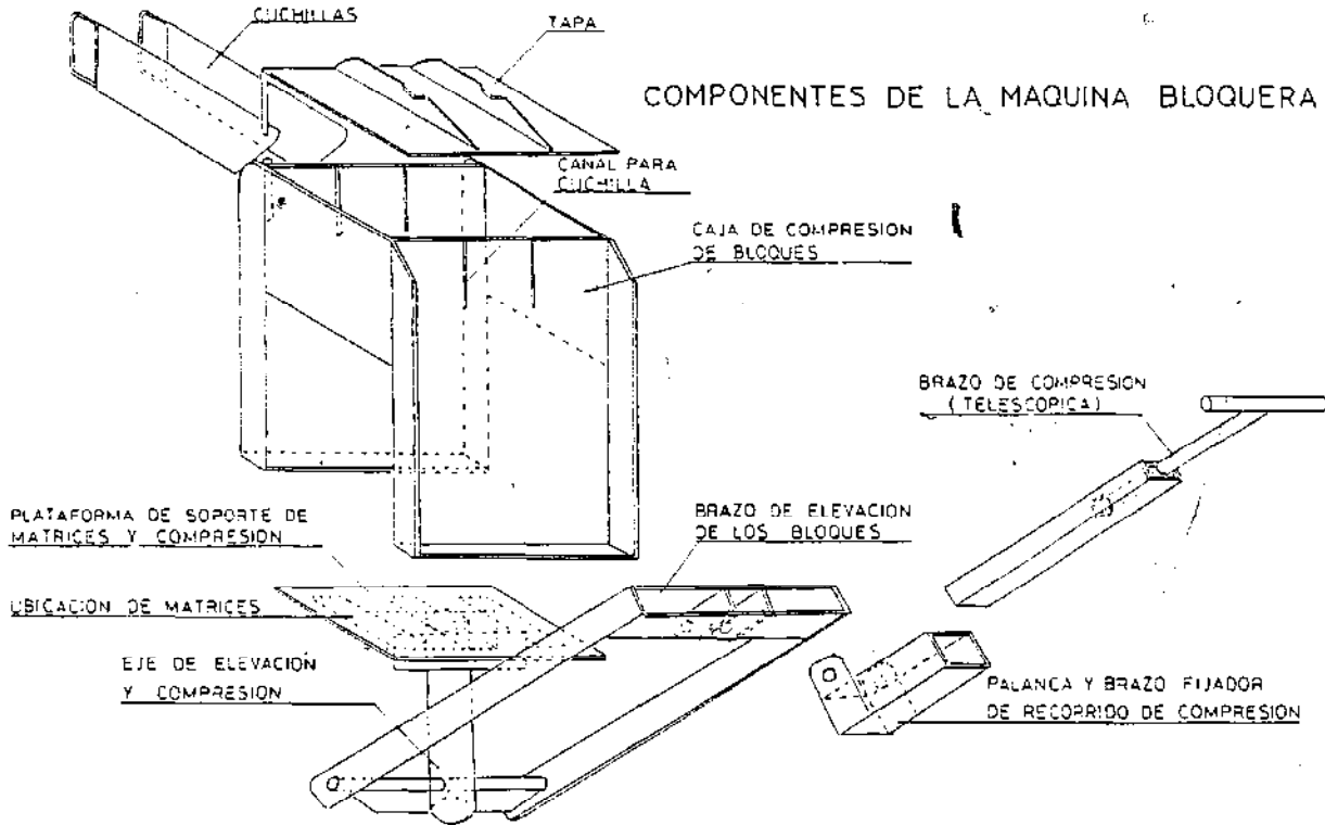
PALANCA Y BRAZO FIJADOR DE RECORRIDO DE COMPRESION
