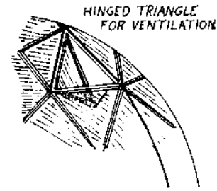
Fig. 4 - Ventilation
