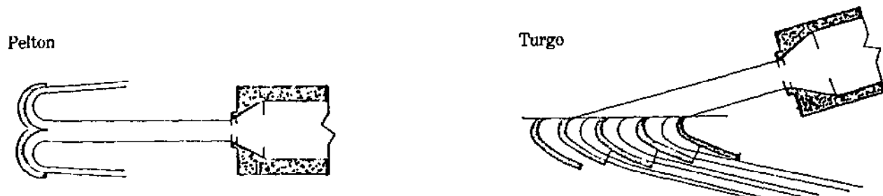
Figura 7b Contraste de las Turbinas Turgo y Pelton. El Chorro en la Turbina Turgo Golpea Continuamente Tres Cubos, Mientras que, en la Pelton, Sólo Golpea Uno. Un efecto Análogo de Incremento de la Velocidad Puede Obtenerse en la Turbina Pelton Añadiendo Uno o Dos Chorro Más. Figure 7b Turgo and Pelton Turbines Contrasted. The Jet on the Turgo Strikes Three Buckets Continuously, Whereas on the Pelton it Strikes Only One. A Similar Speed Increasing Effect Can Be Had On the Pelton by Adding Another Jet or Two.
