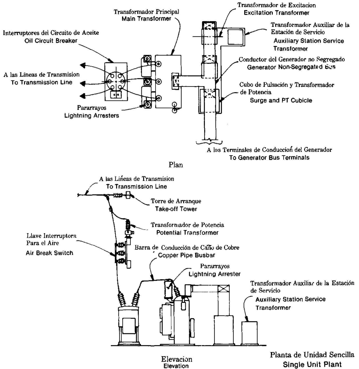
Figura 10 Arreglo típico de un patio de distribución Figure 10 Typical arrangement of a switchyard
