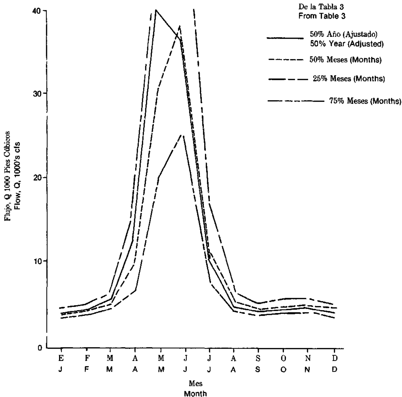
Figura 4. Análisis de los Valores Fluviales Mensuales del 50% del Año Índice y de Curvas de la Duración-Fluvial Mensual
