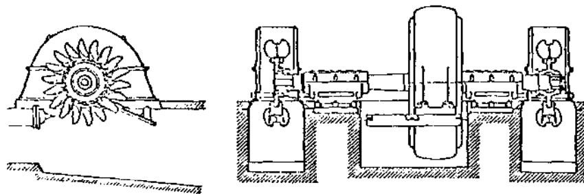
Figura 7a Rueda de Impulsos de Montante Doble Figure 7a Double-Overhung Impulse Wheel
