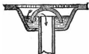
FIG. 221.—Bell Trap.
