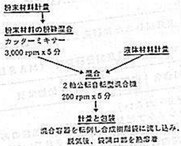
図2：製造方法
