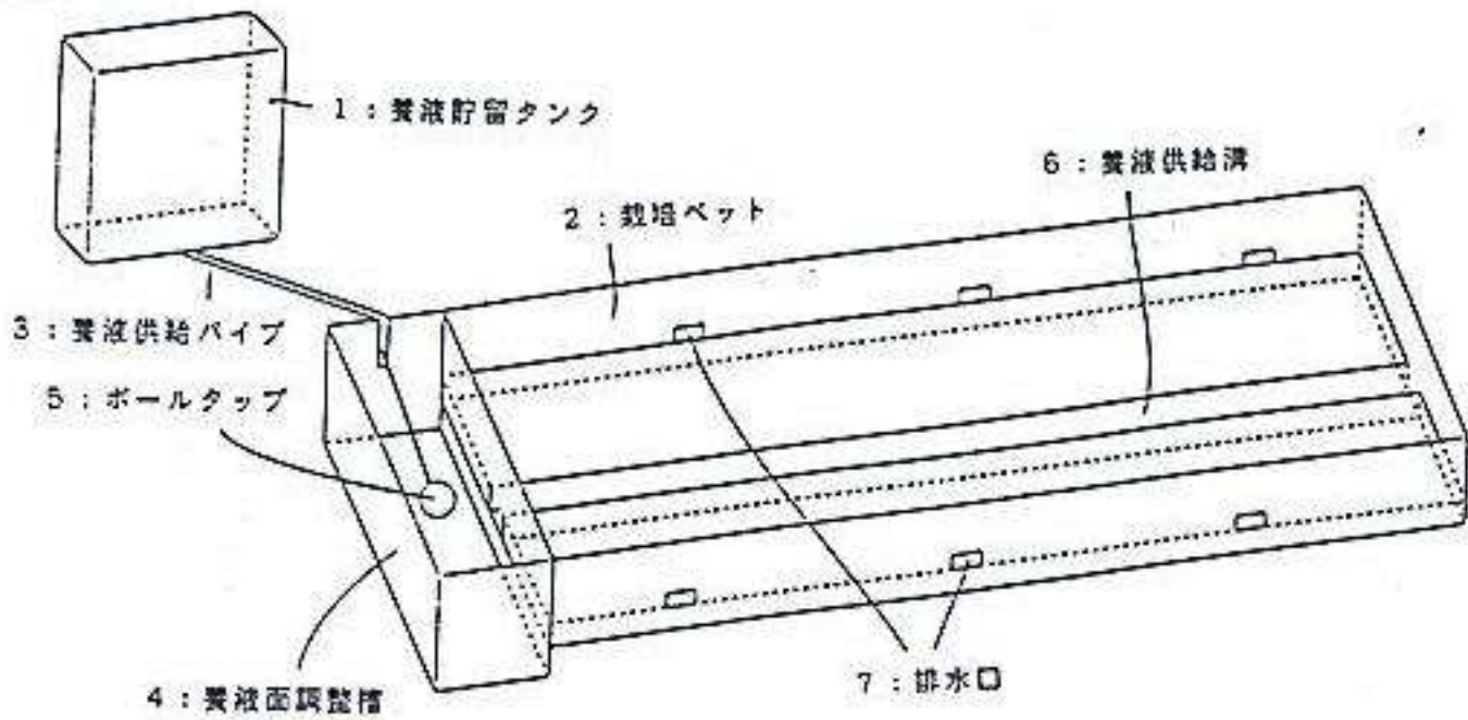
図1 装置概略図
