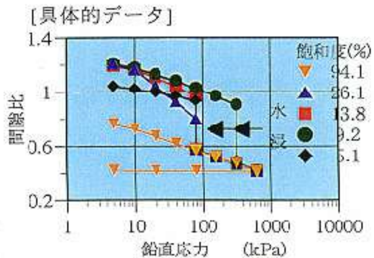
図1 圧密試験結果
