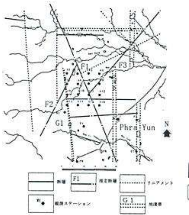
図1 断層分布図
