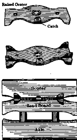
FIG. 144.—Bolster plates.
