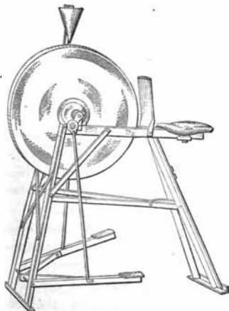
FIG. 111.—Grindstone.
