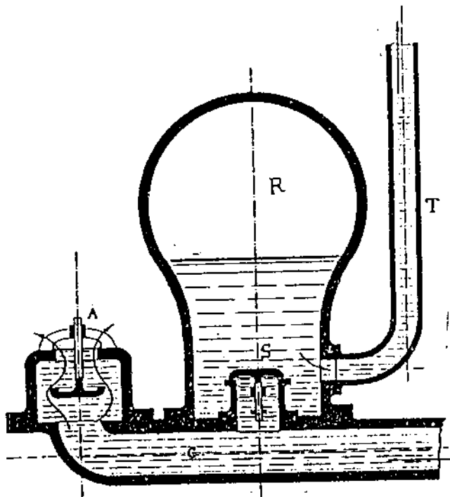
Fig. 2 : Coupe d'un béliet. Période de refondement. Soupape d'arrêl fermée.
