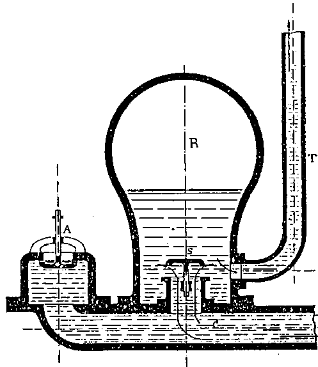
Fig. 3 : Coupe d'un béliet. Période d'écoulement. Soupape d'arrêl ouverte.
