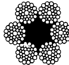
D Cable bent ropes
