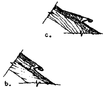
Abb. 4.41 (a, b, c, d, e) Anschlußdetails für Falzdeckung Fig. 4.41 (a, b, c, d, e) Details of sheet metal connections and seams
