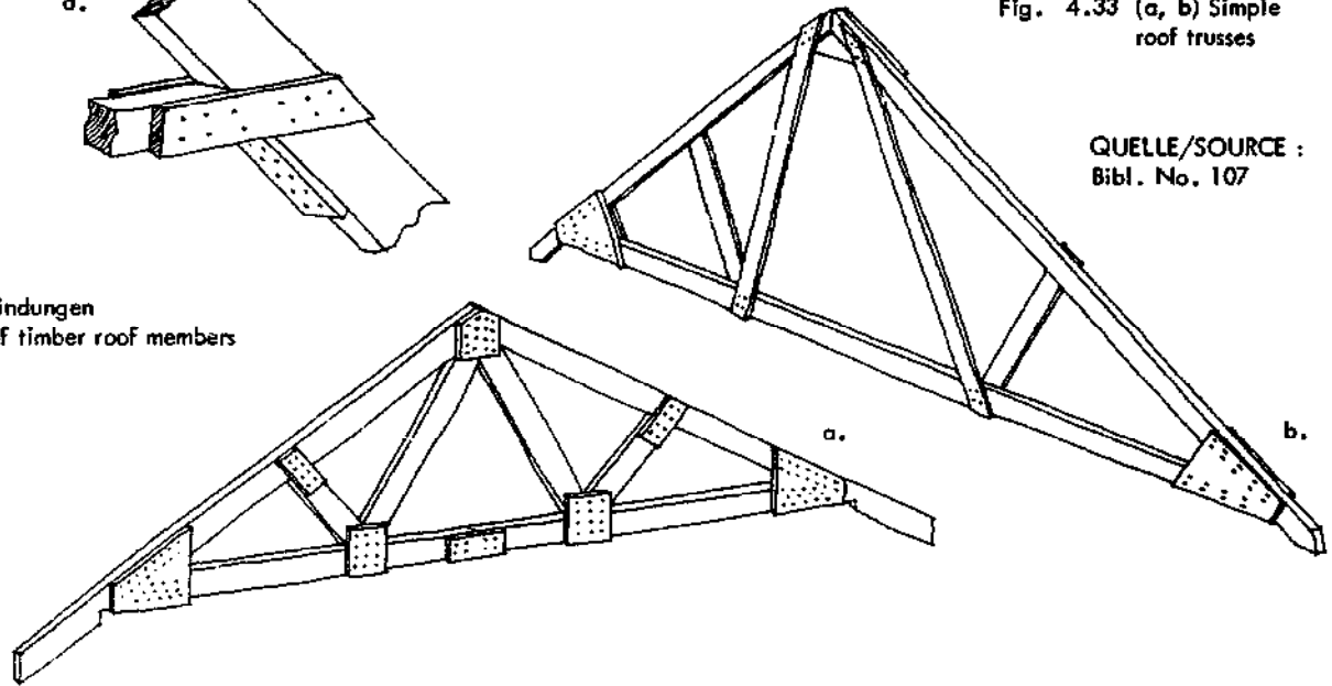
Abb. 4.33 (a, b) Einfache Dachbinder
