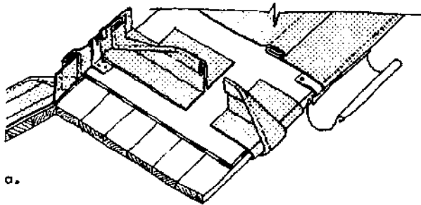
Abb. 4.41 (a, b, c, d, e) Anschlußdetails für Falzdeckung Fig. 4.41 (a, b, c, d, e) Details of sheet metal connections and seams
