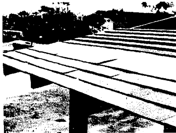
Abb. 4.57 Teilweise montiertes Versuchsdach in Ghana Fig. 4.57 Partially installed test roof in Ghana
