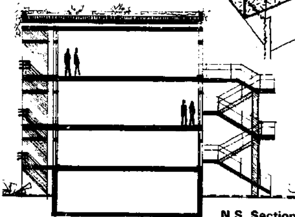
N.S. Section
