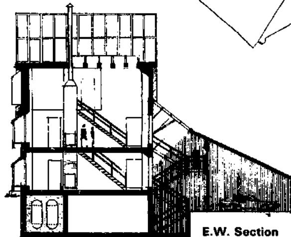
E.W. Section
