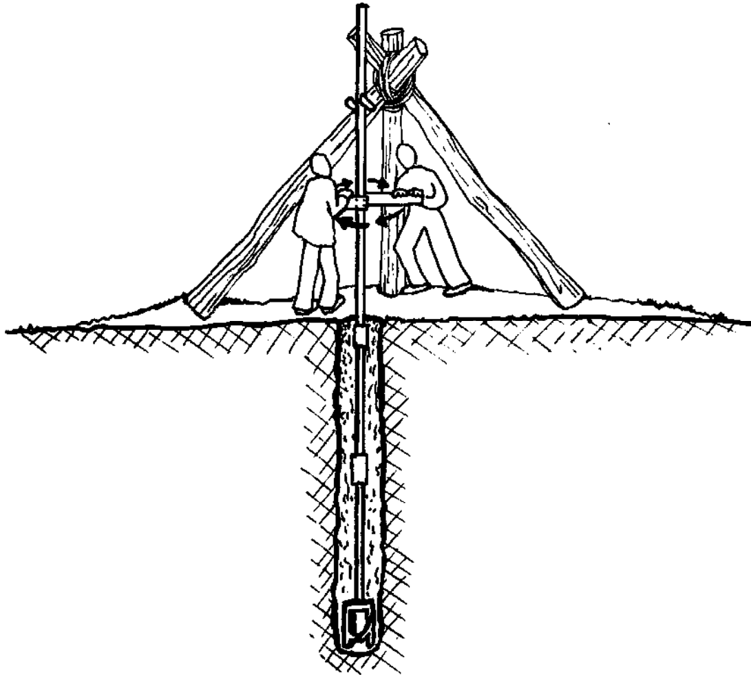
FIG. 12-1. HAND AUGERING
