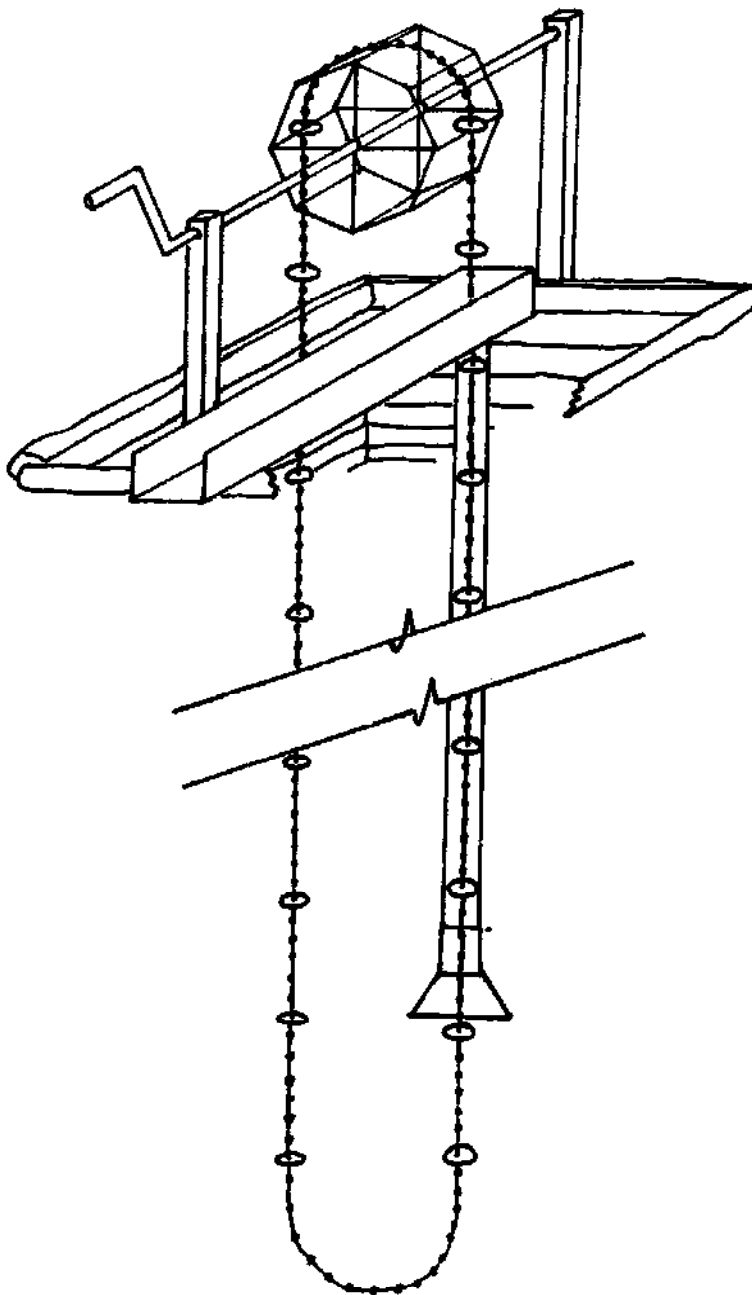
FIG. VII-12. CHAIN PUMP
