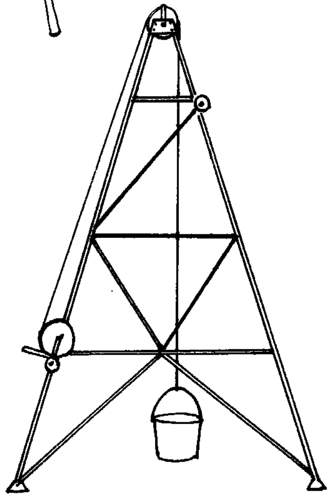
FIG. 5-6. HEADFRAME
