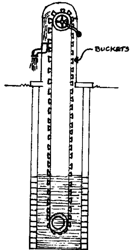
FIG. VII-11. BUCKET PUMP
