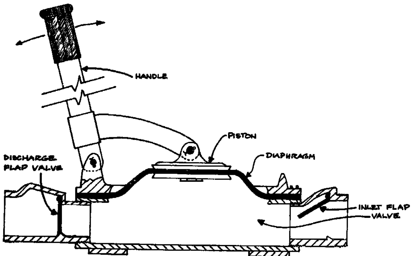
FIG. VII-9. DIAPHRAGM PUMP
