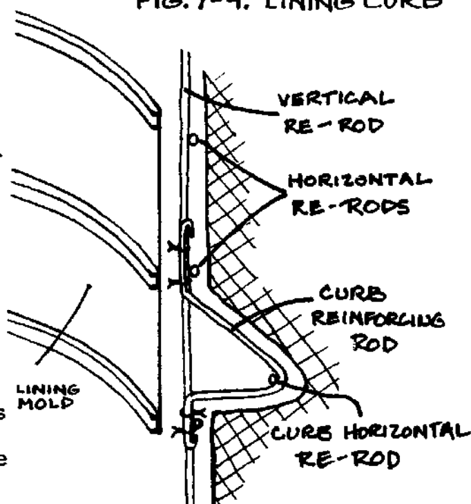
FIG. 7-4. LINING CURB
