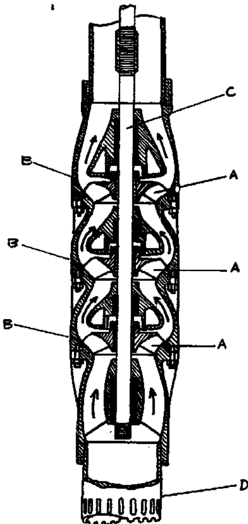
FIG. VII-14. TURBINE PUMP
