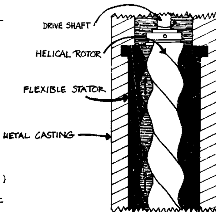
FIG. VII-10. HELICAL ROTOR PUMPING UNIT
