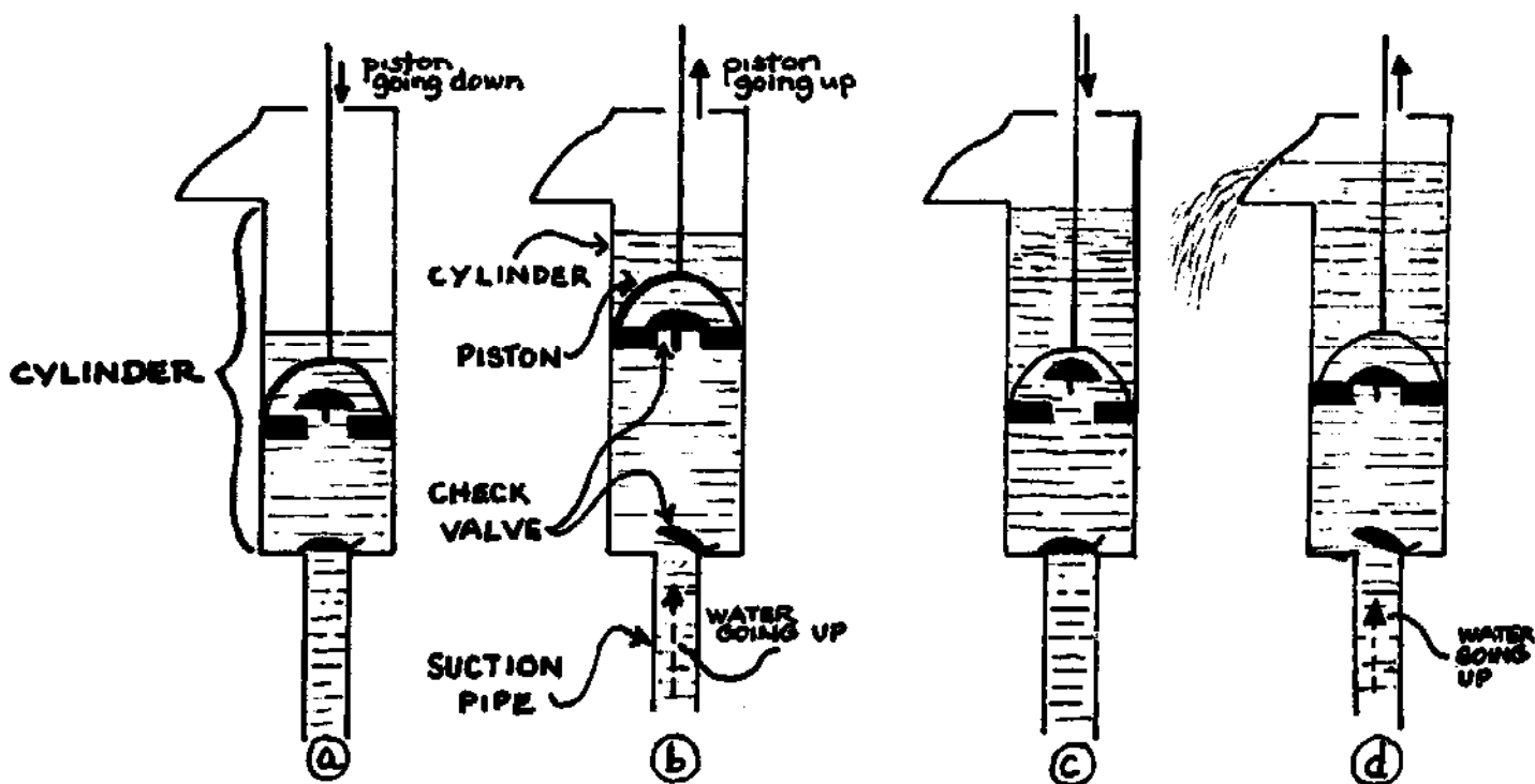
FIG. VII-1. PUMP ACTION
