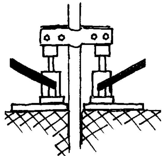
FIG. 14-11. JACK PIPE UP
