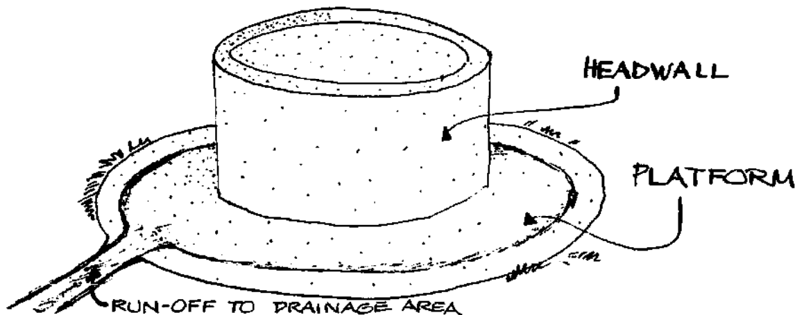
FIG. 3-7. TOP SECTION
