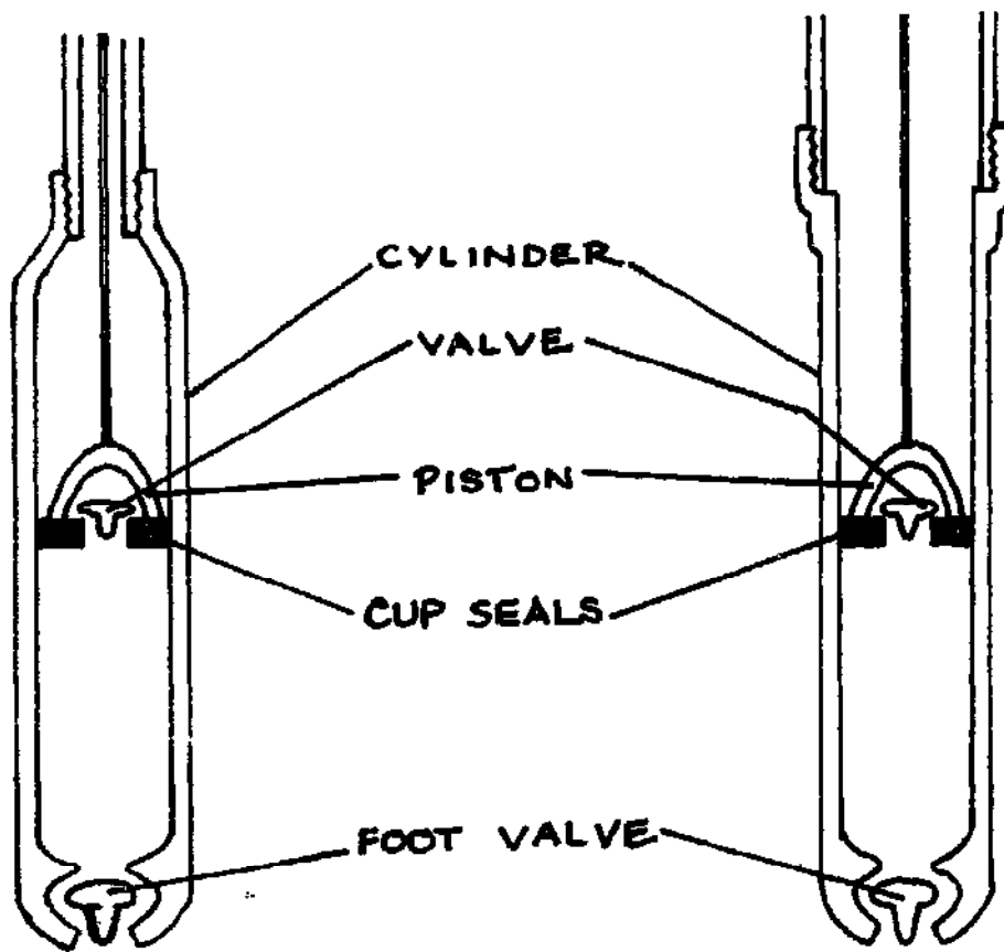
FIG. VII-6. EXTRACTABLE CYLINDER
