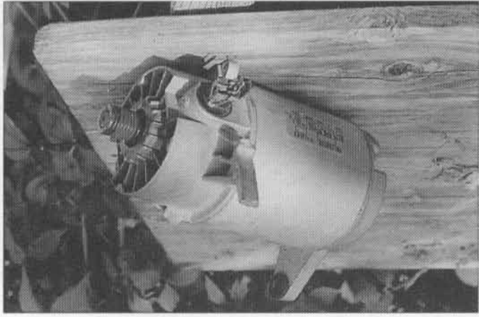
Die häufigere Dauermagnetmotor-Sorte (Polymotor Italiana): Dauermagnete innen gut sichtbar. - Motor von außen. (leider hat der Schrottarbeiter die Halterung abgebrochen)
